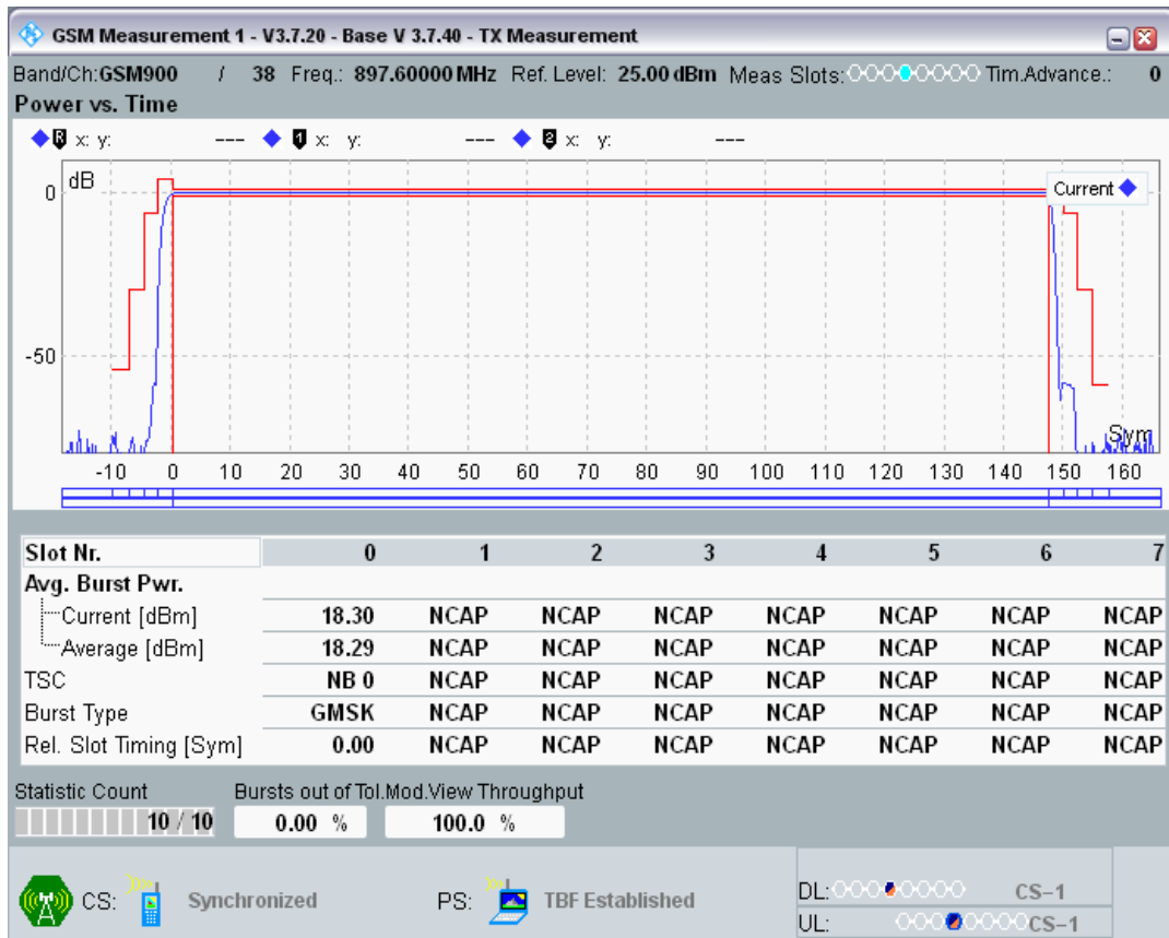
GPRS900 Channel=38 Gamma=5;5;5;5
