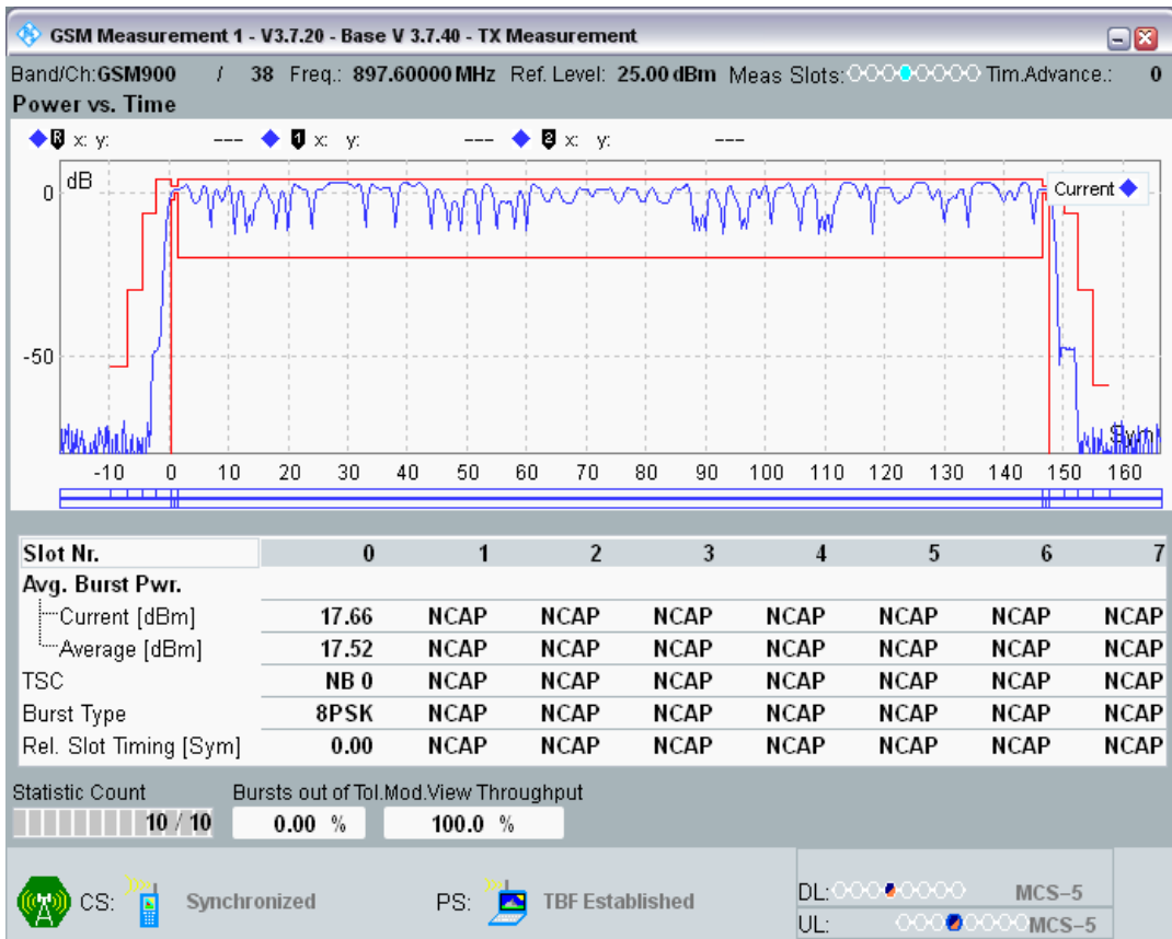
EGPRS900 Channel=38 Gamma=11;11;11;11
