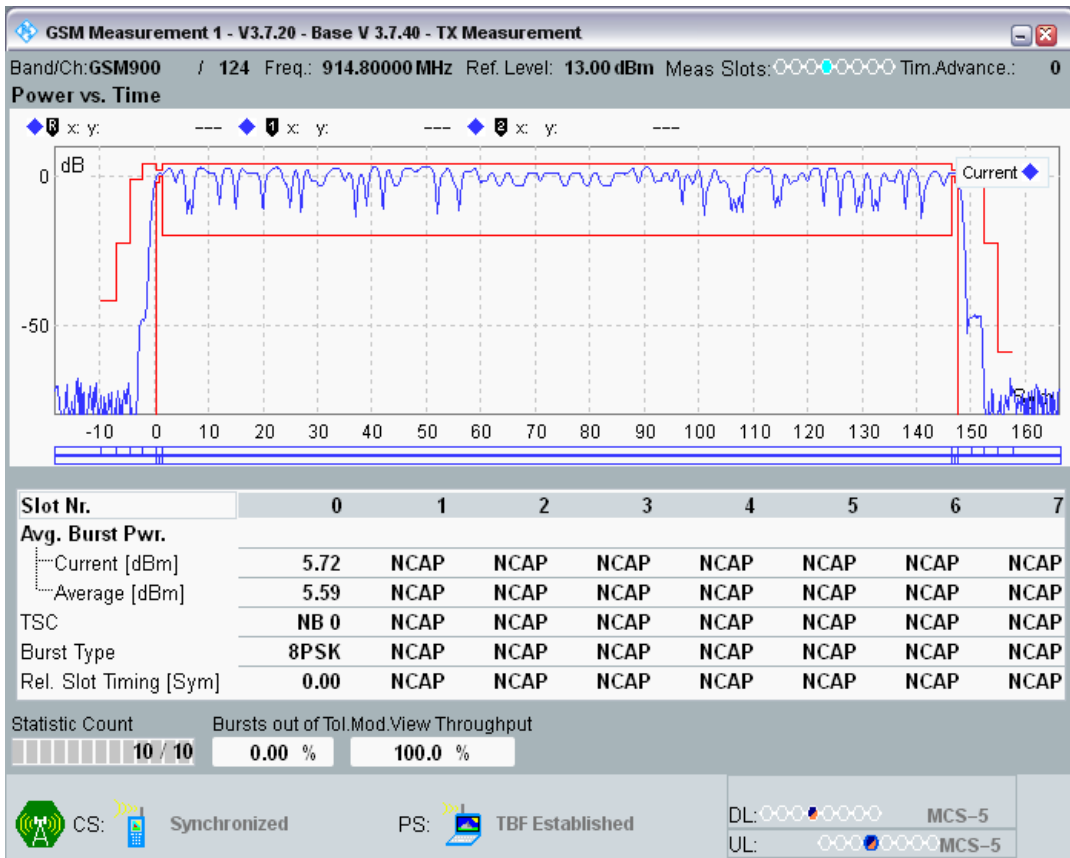
EGPRS900 Channel=124 Gamma=17;17;17;17
