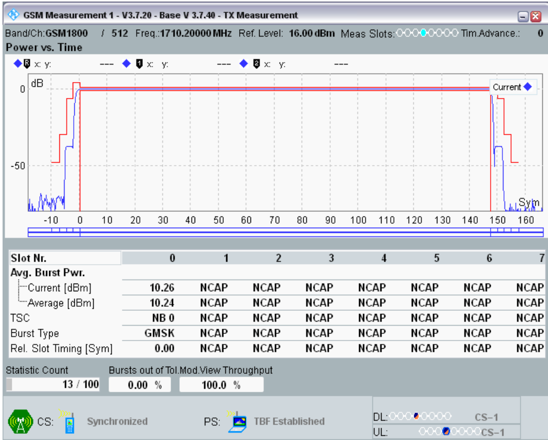
GPRS1800 Channel=512 Gamma=9;9;9
