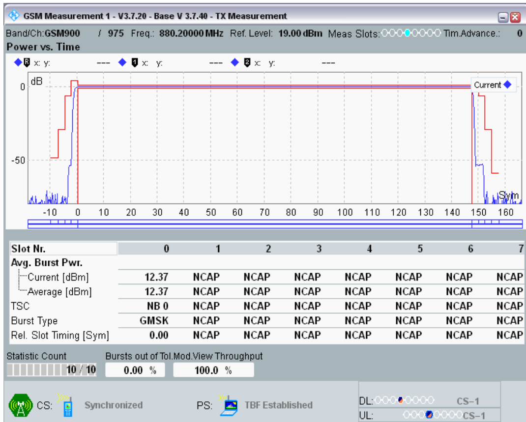
GPRS900 Channel=975 Gamma=12;12;12;12
