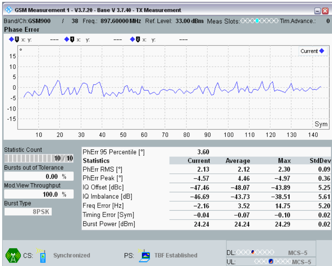
EGPRS900 Channel=38 Gamma=6;6;6;6 TU50 @Sens5
