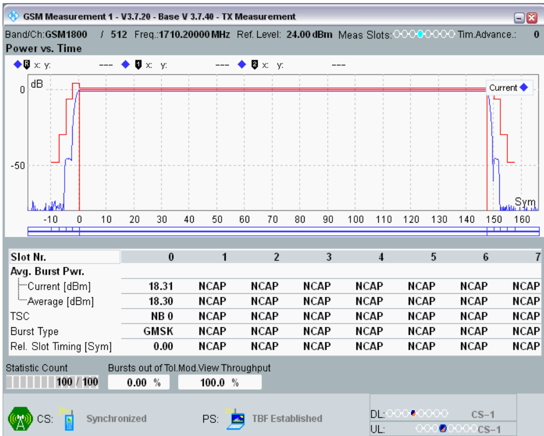
GPRS1800 Channel=512 Gamma=8;8;8
