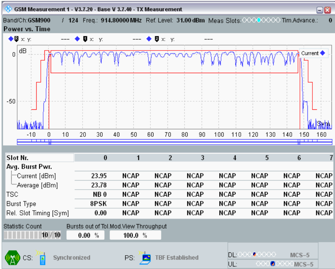
EGPRS900 Channel=124 Gamma=9;9;9;9
