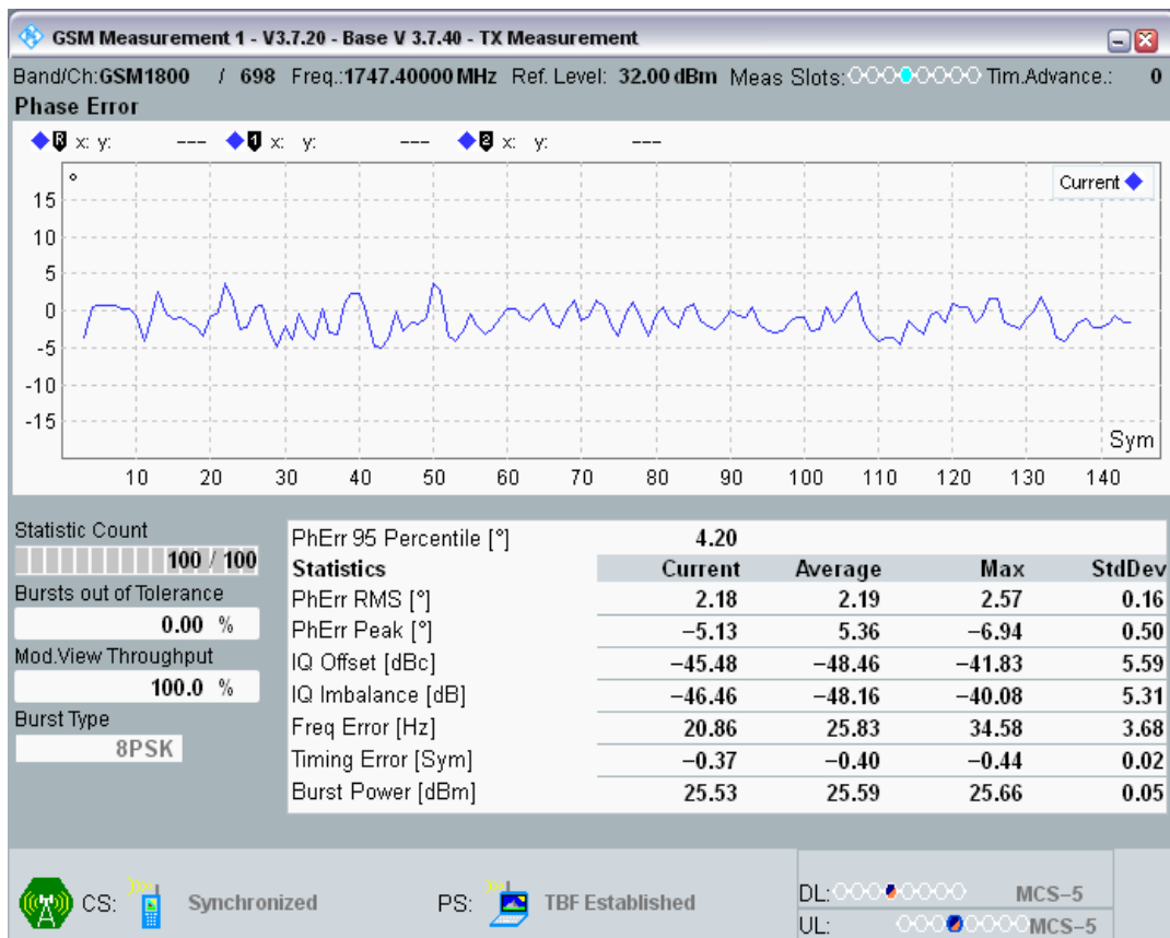
EGPRS1800 Channel=698 Gamma=5;5;5;5 TU5 @Sens1
