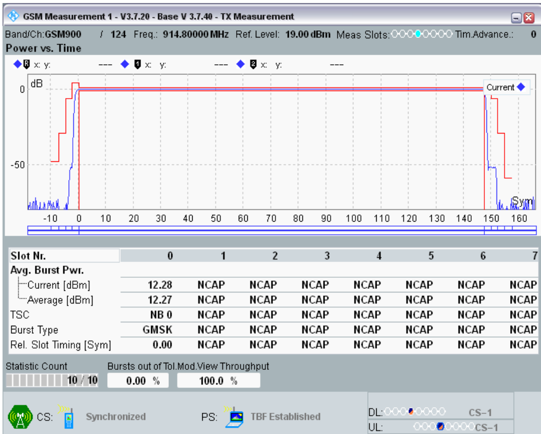
GPRS900 Channel=124 Gamma=12;12;12;12
