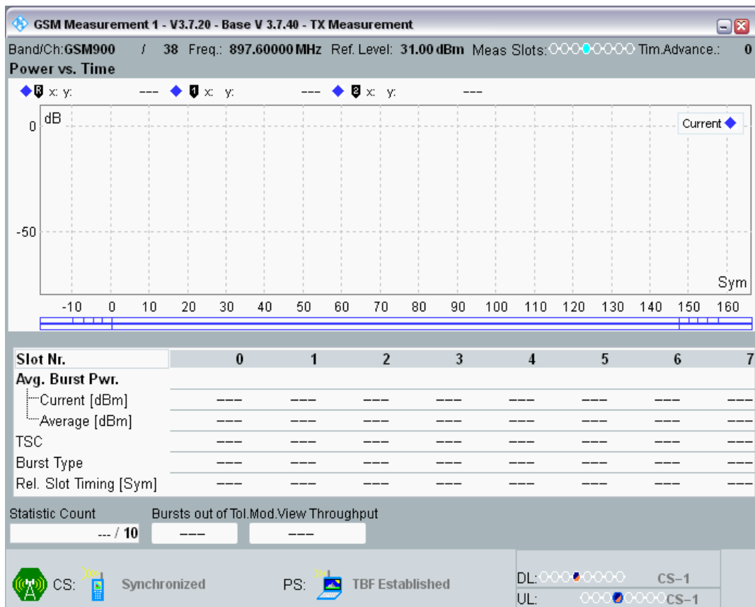
GPRS900 Channel=38 Gamma=15;15;15
