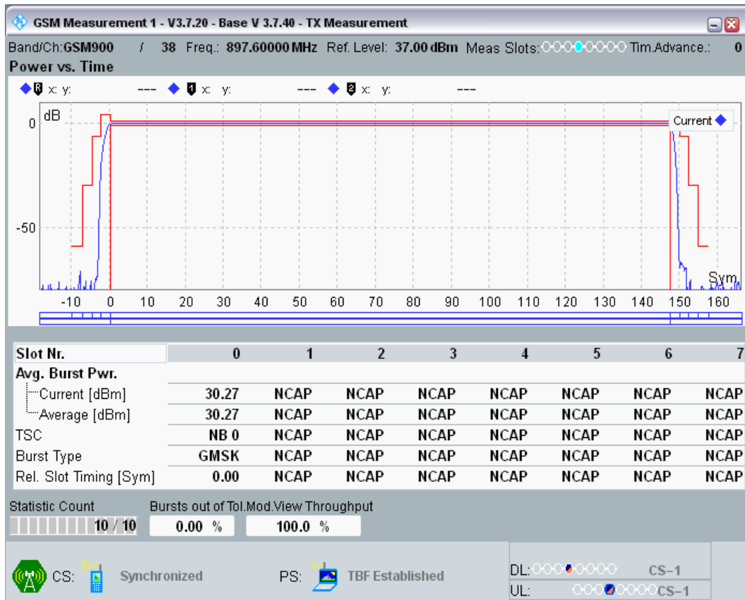
GPRS900 Channel=38 Gamma=6;6;6
