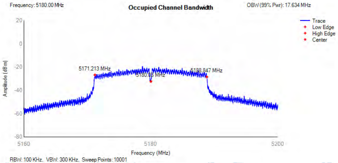
OBW NVNT 802.11n(HT20) 5180MHz
