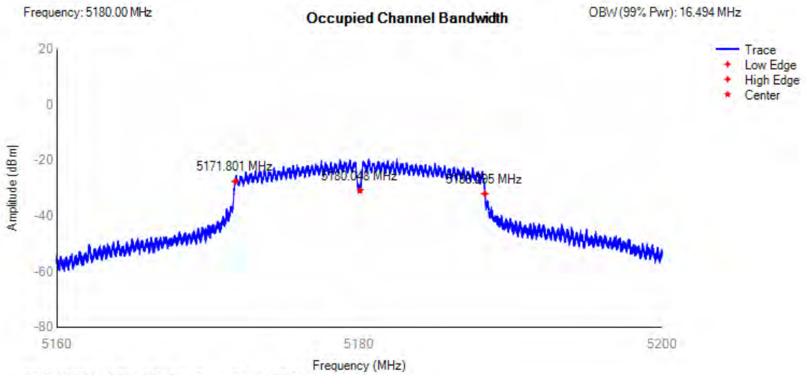
OBW NVNT 802.11n(HT20) 5180MHz
