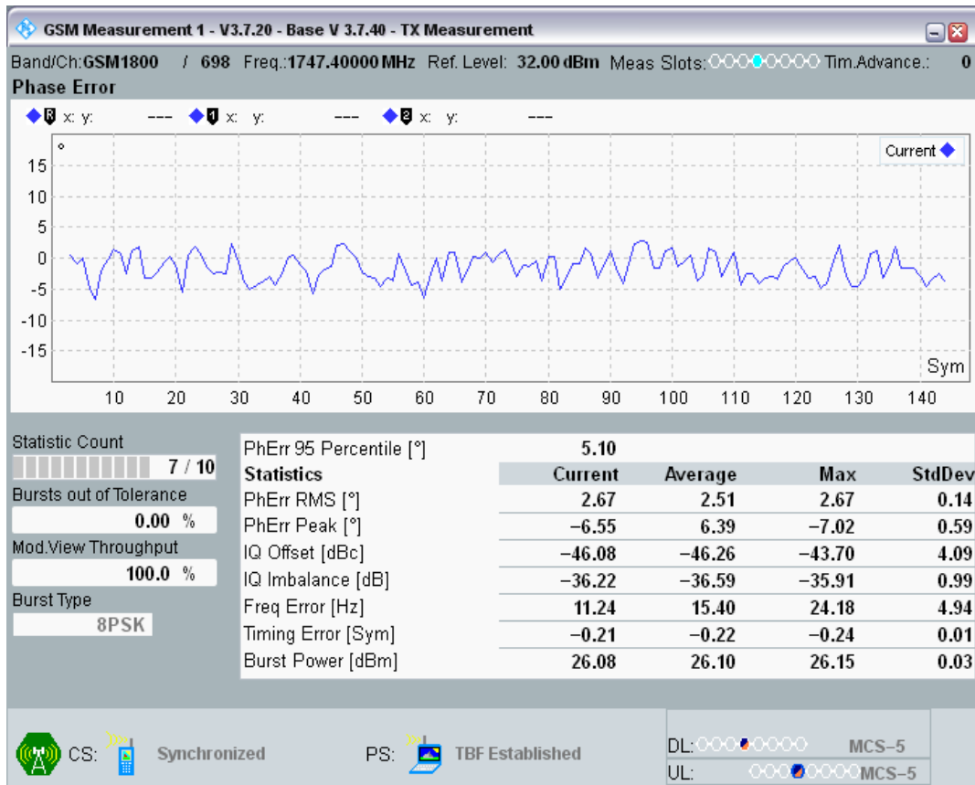
EGPRS1800 Channel=698 Gamma=5;5;5;5 TU3 @8
