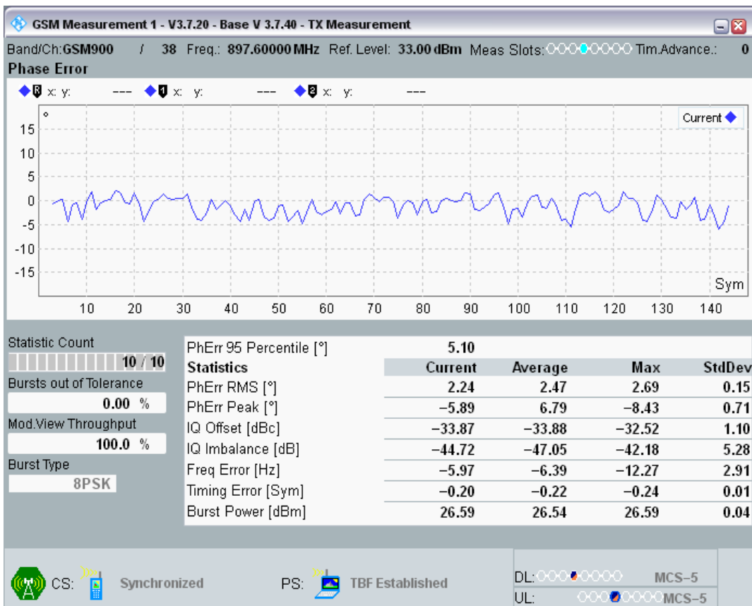
EGPRS900 Channel=38 Gamma=6;6;6;6 TU3 @10
