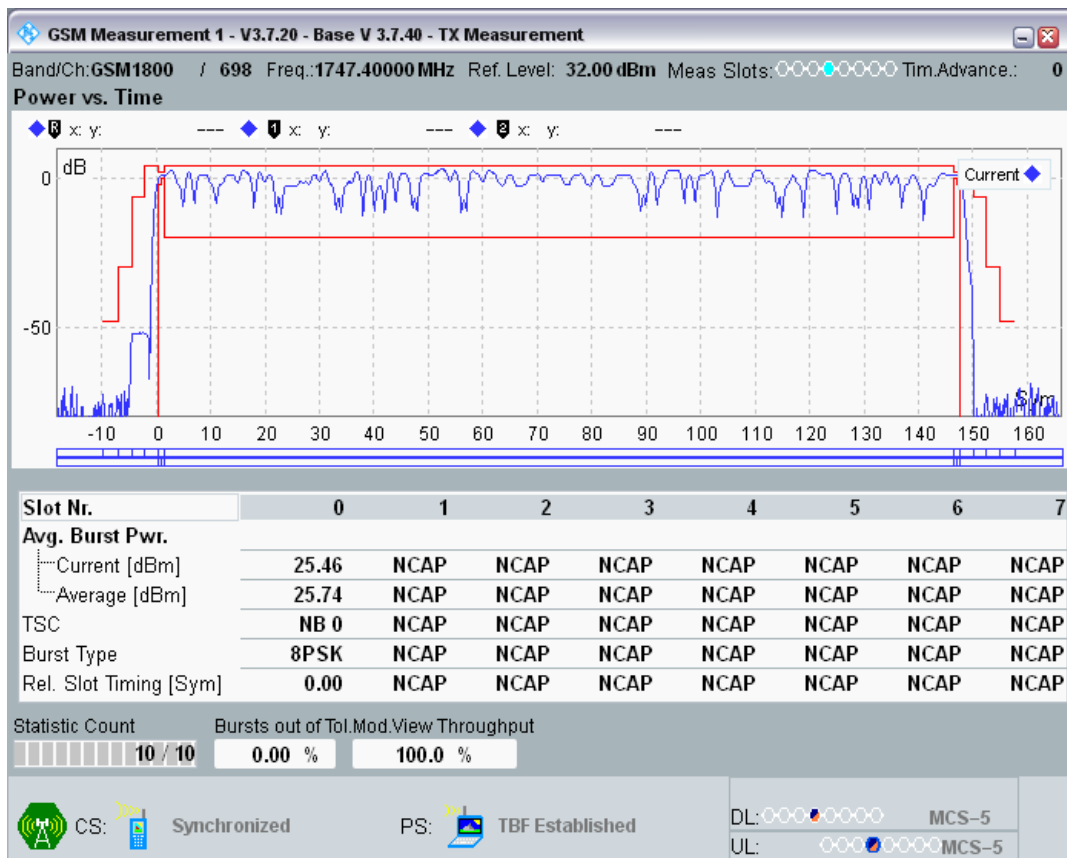
EGPRS1800 Channel=698 Gamma=6;6;6
