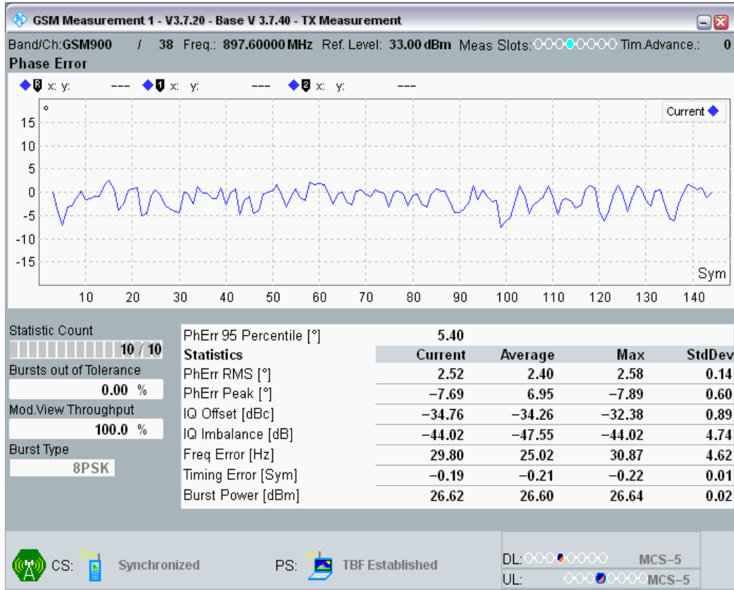
EGPRS900 Channel=38 Gamma=6;6;6;6 RA250 @Sens3
