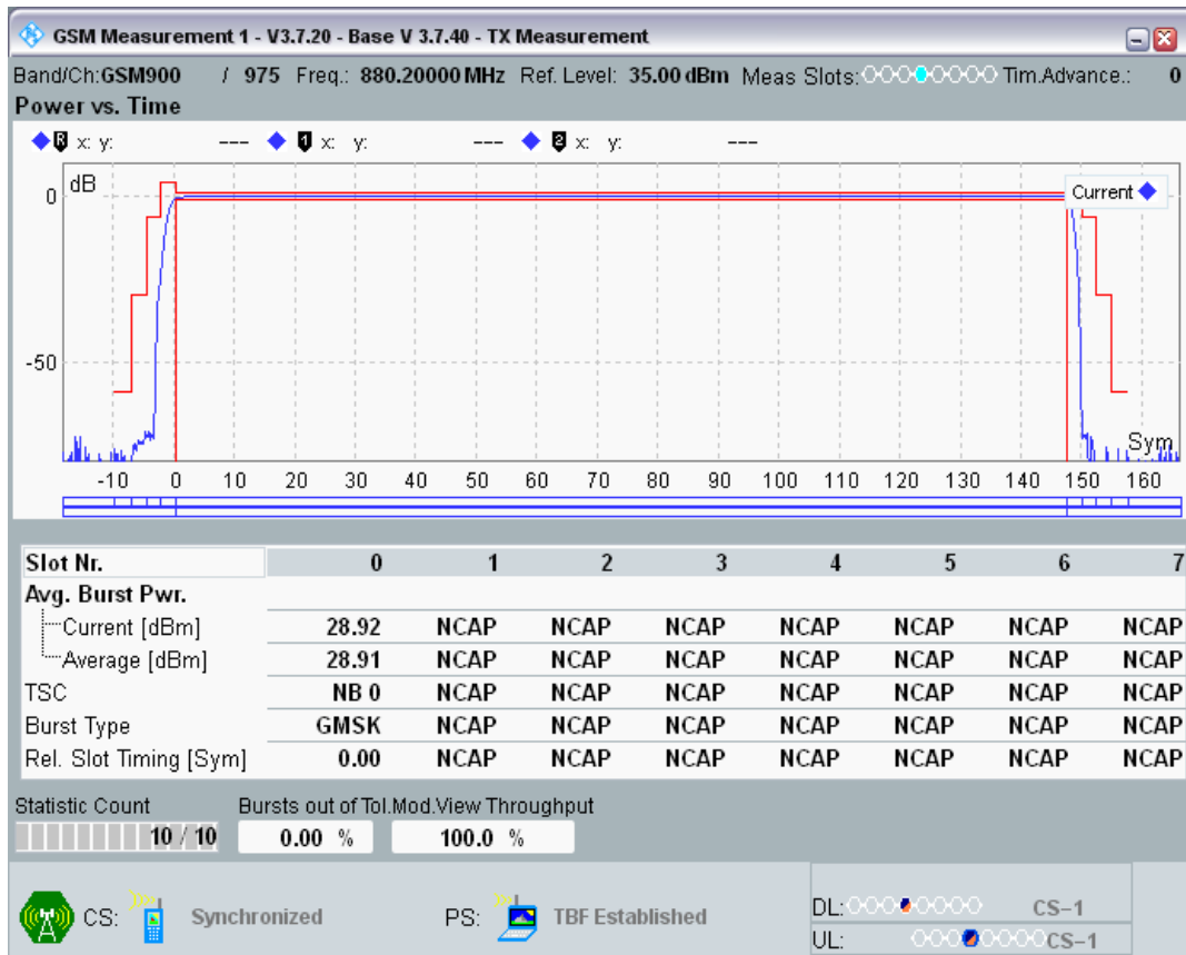
GPRS900 Channel=975 Gamma=6;6;6;6
