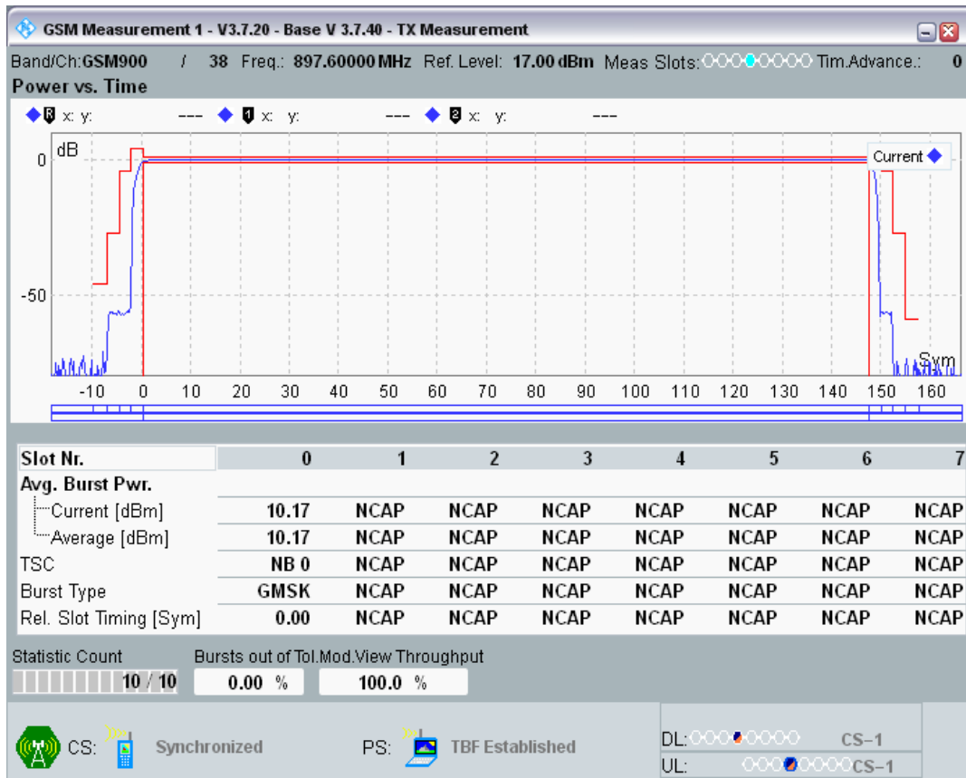
GPRS900 Channel=38 Gamma=15;15;15;15
