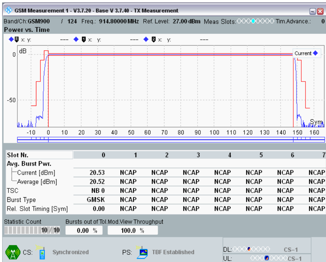
GPRS900 Channel=124 Gamma=11;11;11;11
