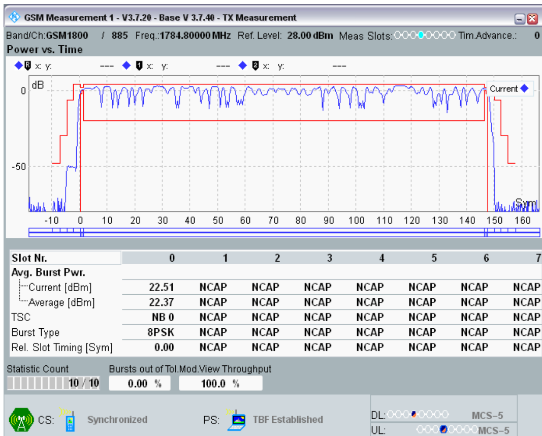
EGPRS1800 Channel=885 Gamma=8;8;8
