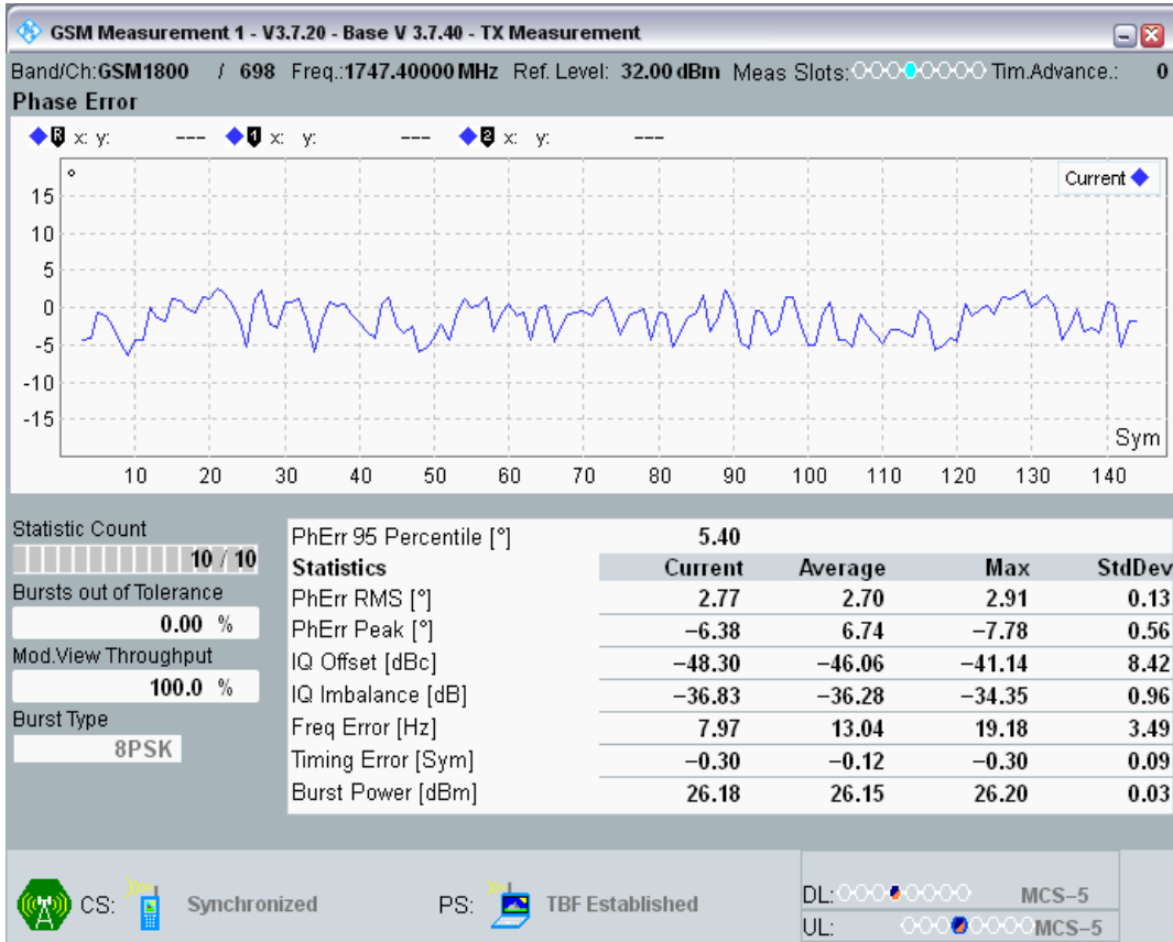
EGPRS1800 Channel=698 Gamma=5;5;5;5 HT100 @Connect
