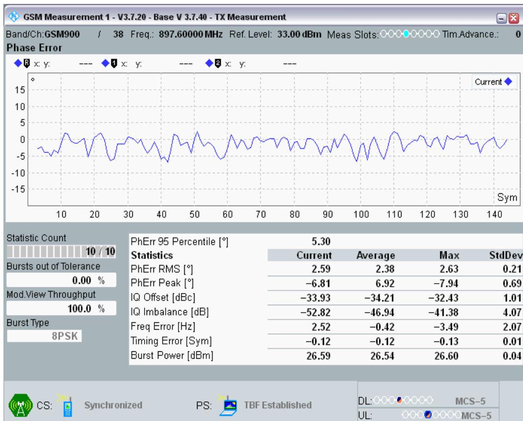
EGPRS900 Channel=38 Gamma=6;6;6;6 TU3 @3
