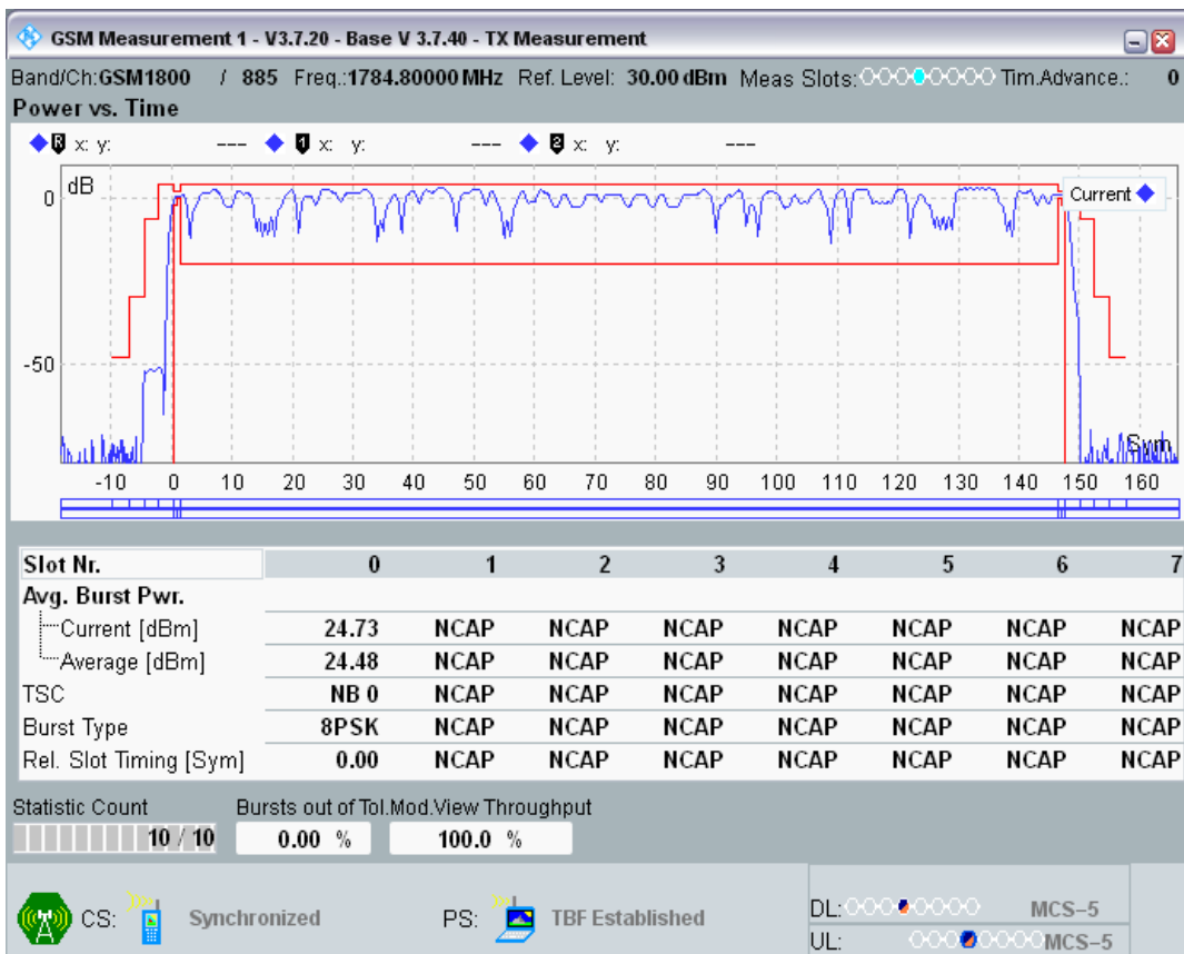
EGPRS1800 Channel=885 Gamma=5;5;5
