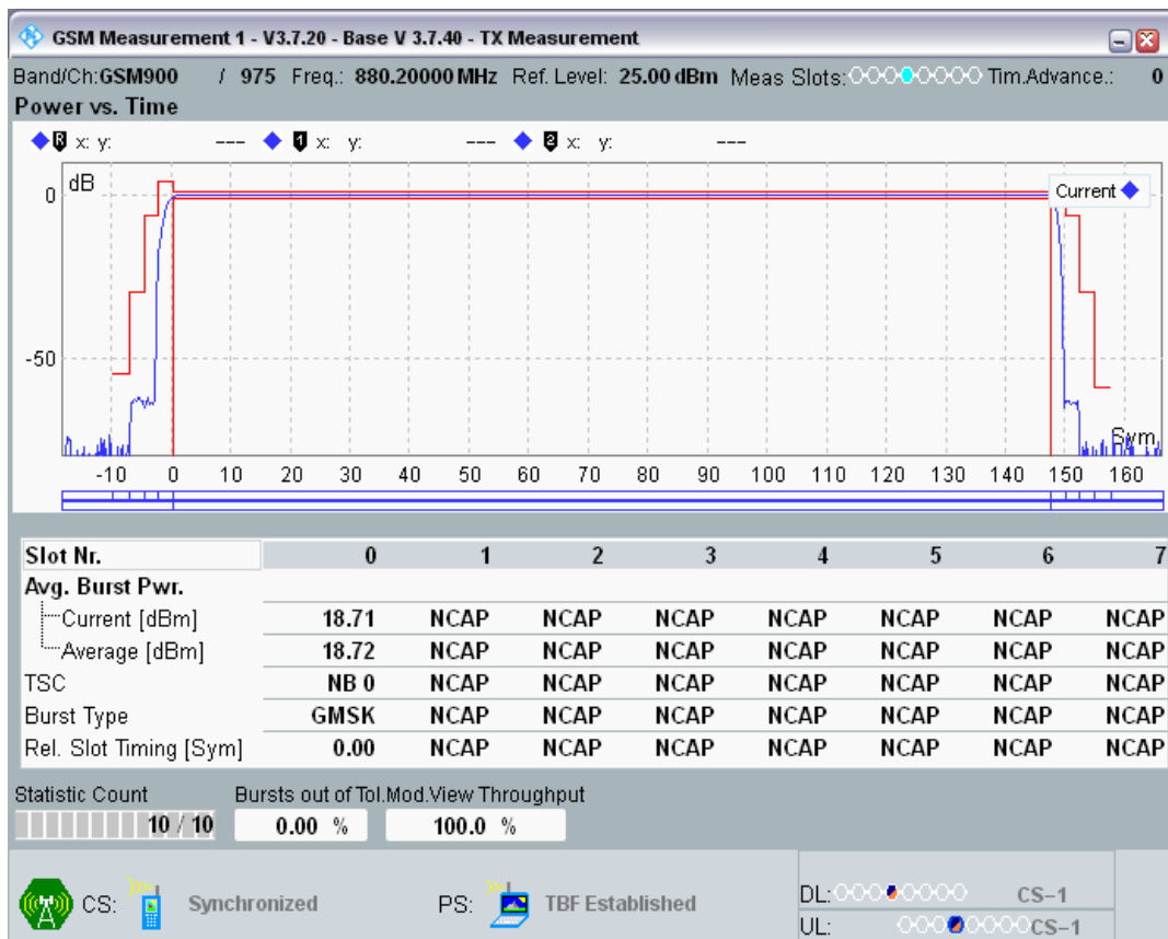
GPRS900 Channel=975 Gamma=11;11;11;11
