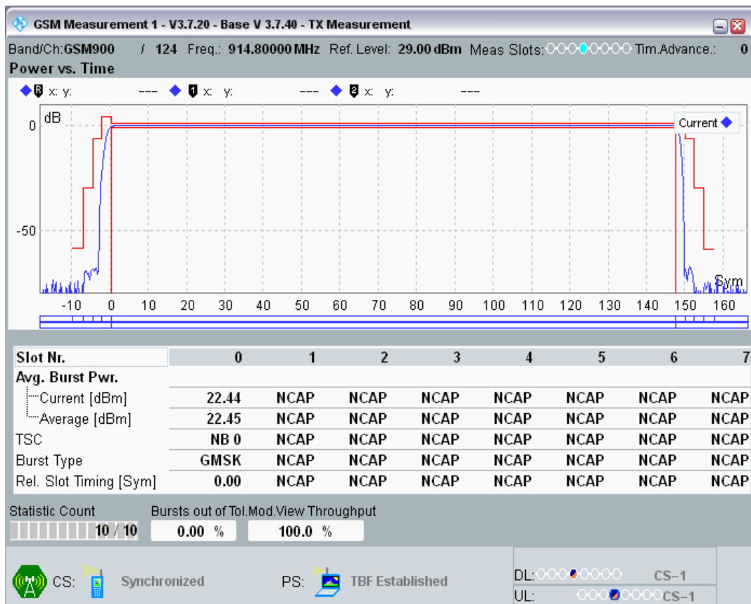
GPRS900 Channel=124 Gamma=10;10;10;10
