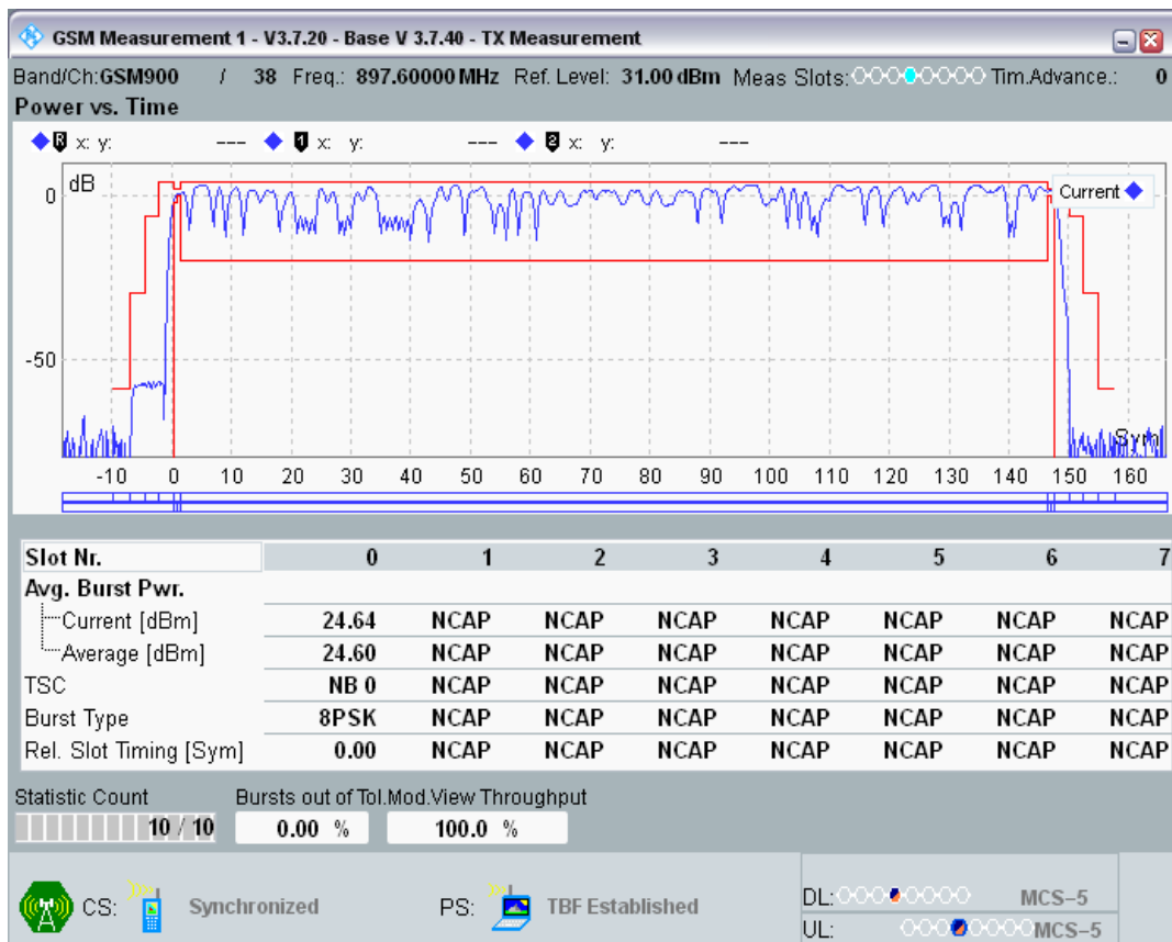
EGPRS900 Channel=38 Gamma=6;6;6
