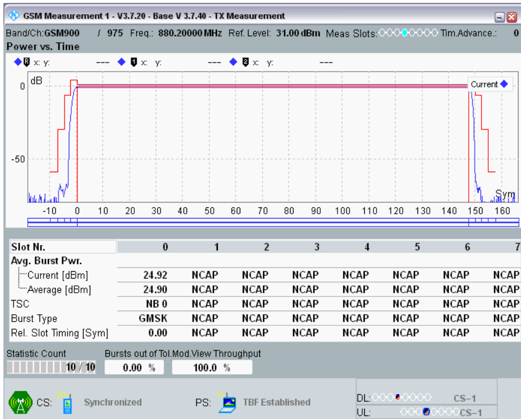
GPRS900 Channel=975 Gamma=8;8;8;8
