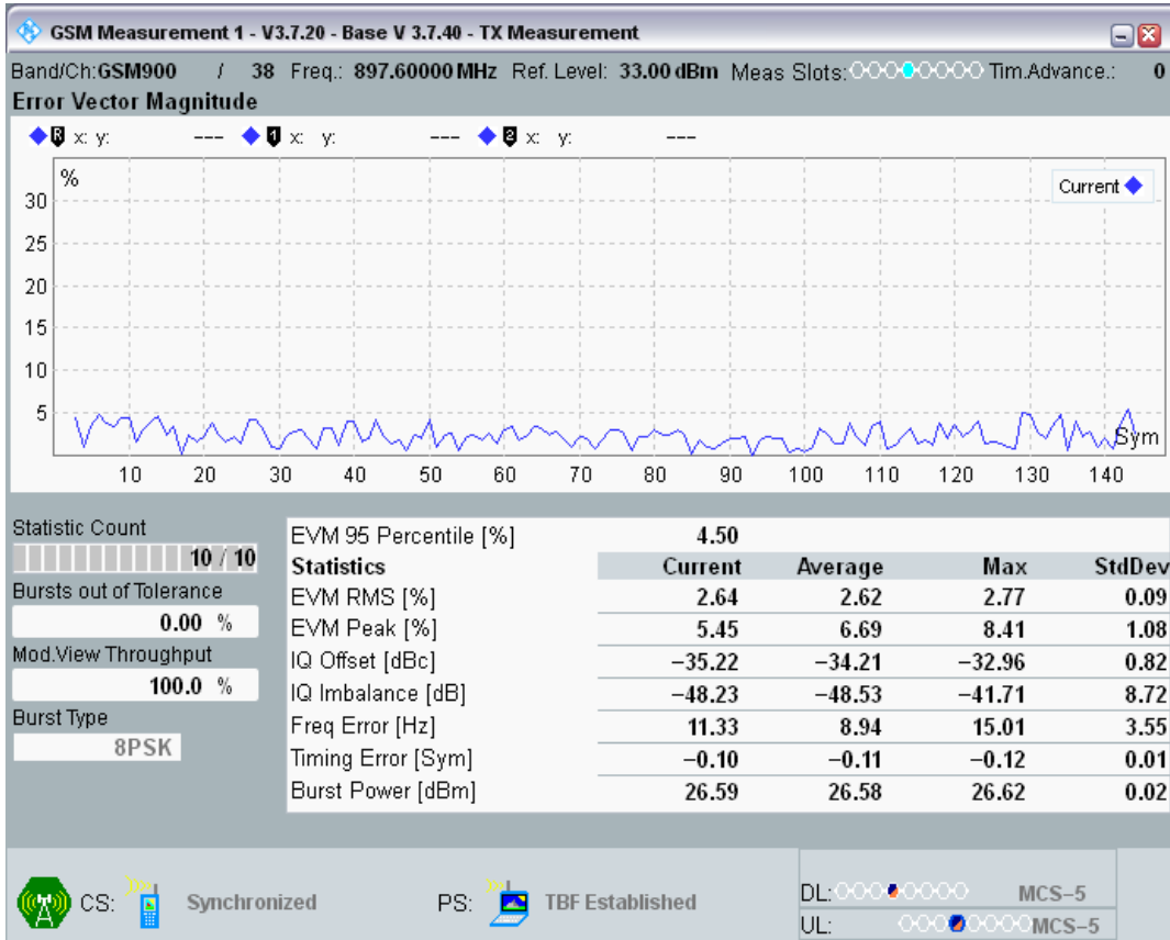
EGPRS900 Channel=38 Gamma=6;6;6;6 HT100 @Sens1
