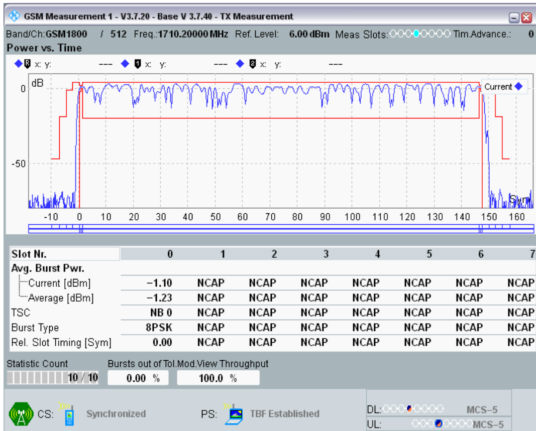
EGPRS1800 Channel=698 Gamma=5;5;5
