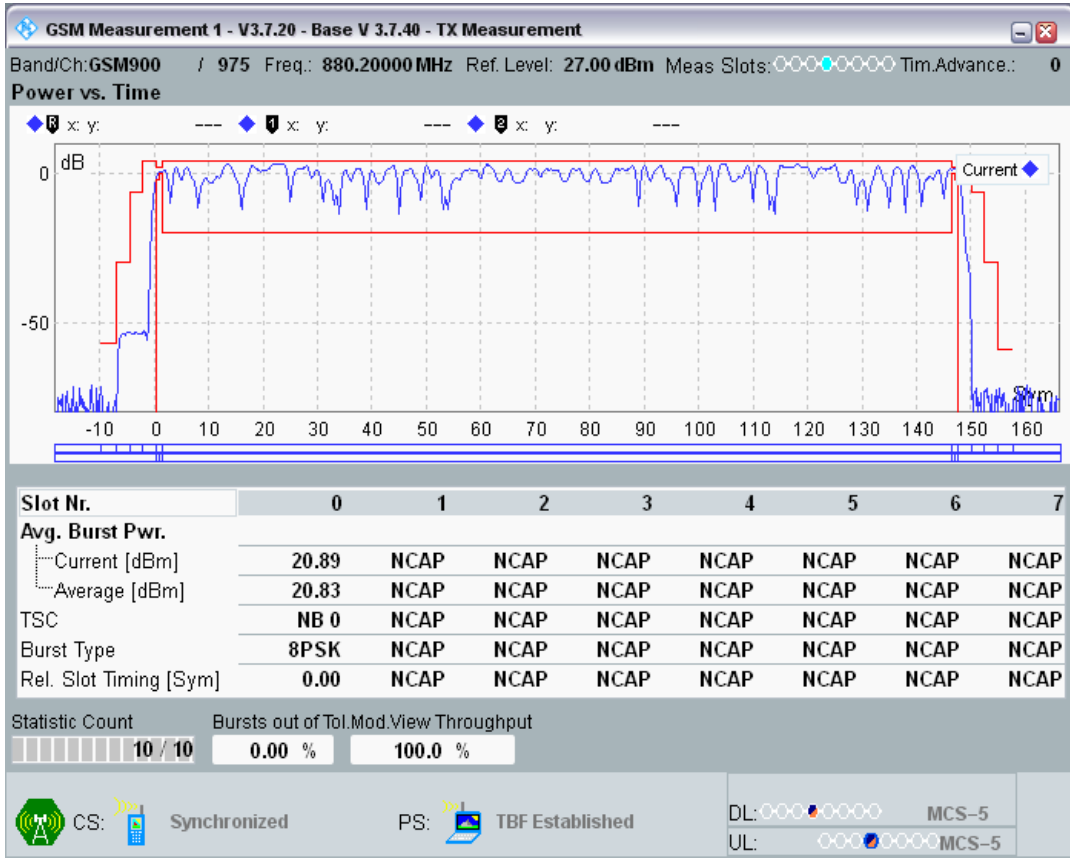
EGPRS900 Channel=975 Gamma=10;10;10;10
