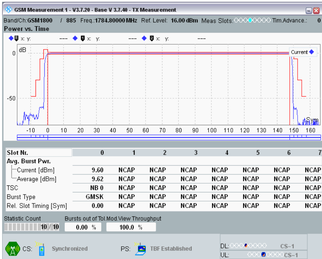
GPRS1800 Channel=885 Gamma=14;14;14;14
