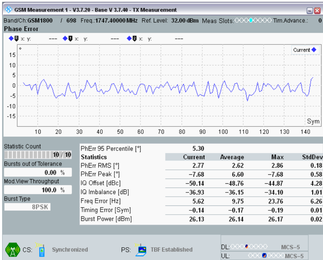
EGPRS1800 Channel=698 Gamma=5;5;5;5 HT100 @Sens4
