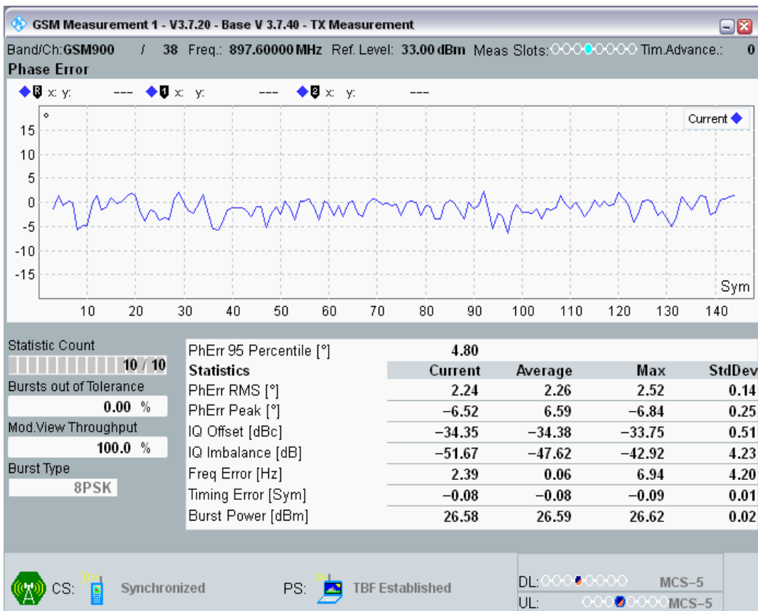
EGPRS900 Channel=38 Gamma=6;6;6;6 HT100 @Sens3
