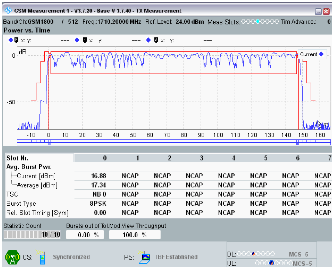
EGPRS1800 Channel=512 Gamma=10;10;10;10
