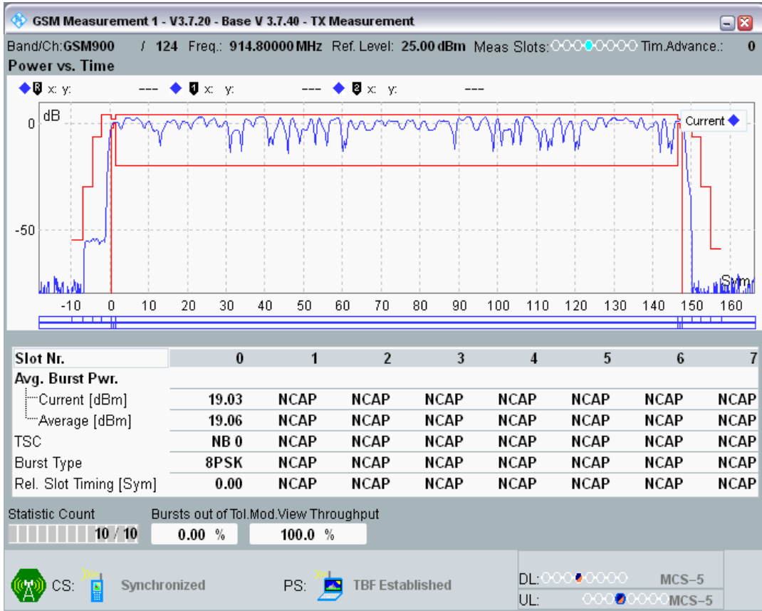
EGPRS900 Channel=124 Gamma=12;12;12;12
