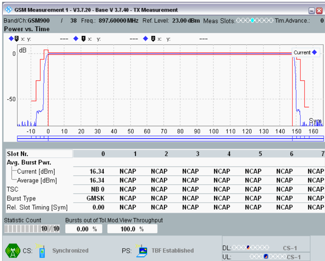
GPRS900 Channel=38 Gamma=13;13;13;13
