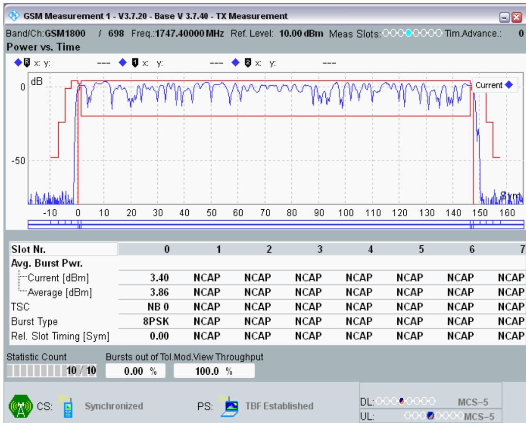
EGPRS1800 Channel=698 Gamma=17;17;17;17
