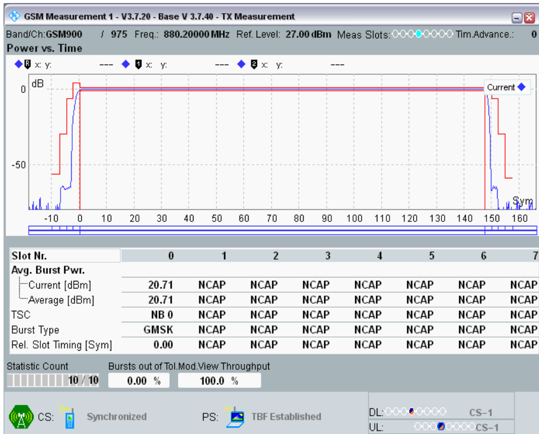
GPRS900 Channel=975 Gamma=10;10;10;10
