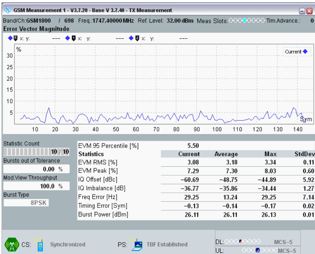
EGPRS1800 Channel=698 Gamma=5;5;5;5 HT100 @Sens2
