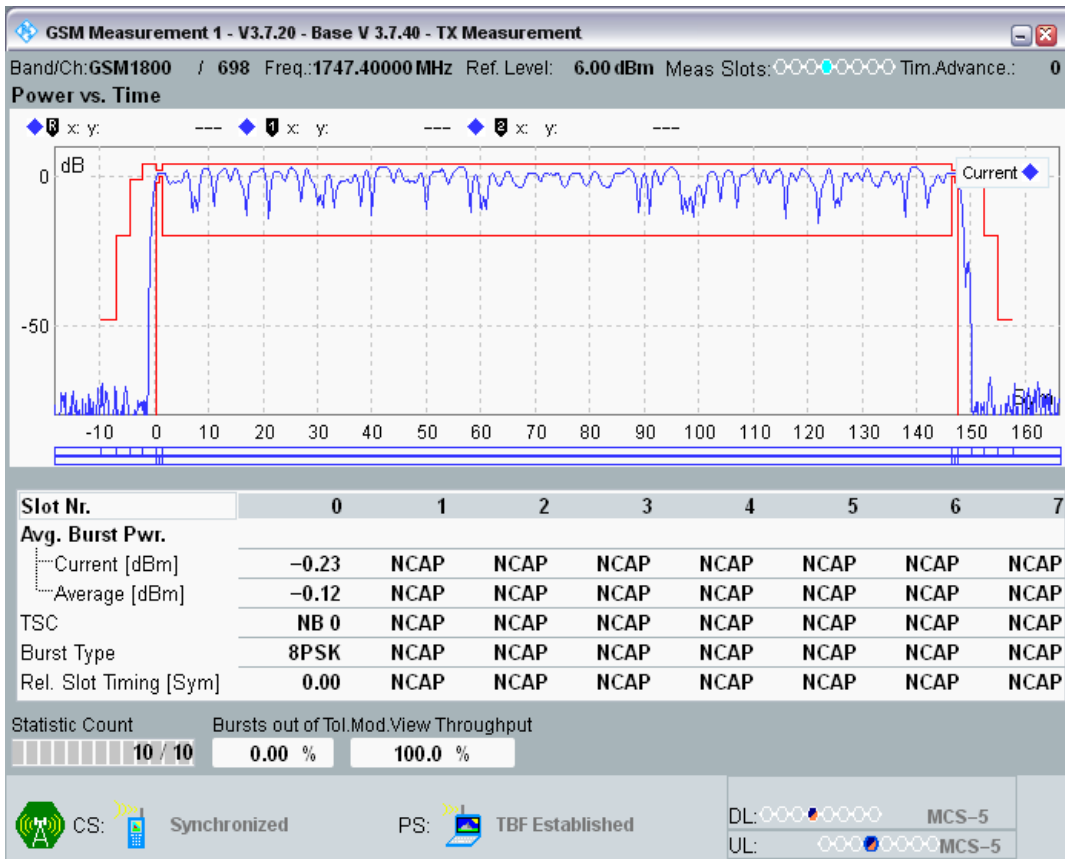
EGPRS1800 Channel=885 Gamma=6;6;6
