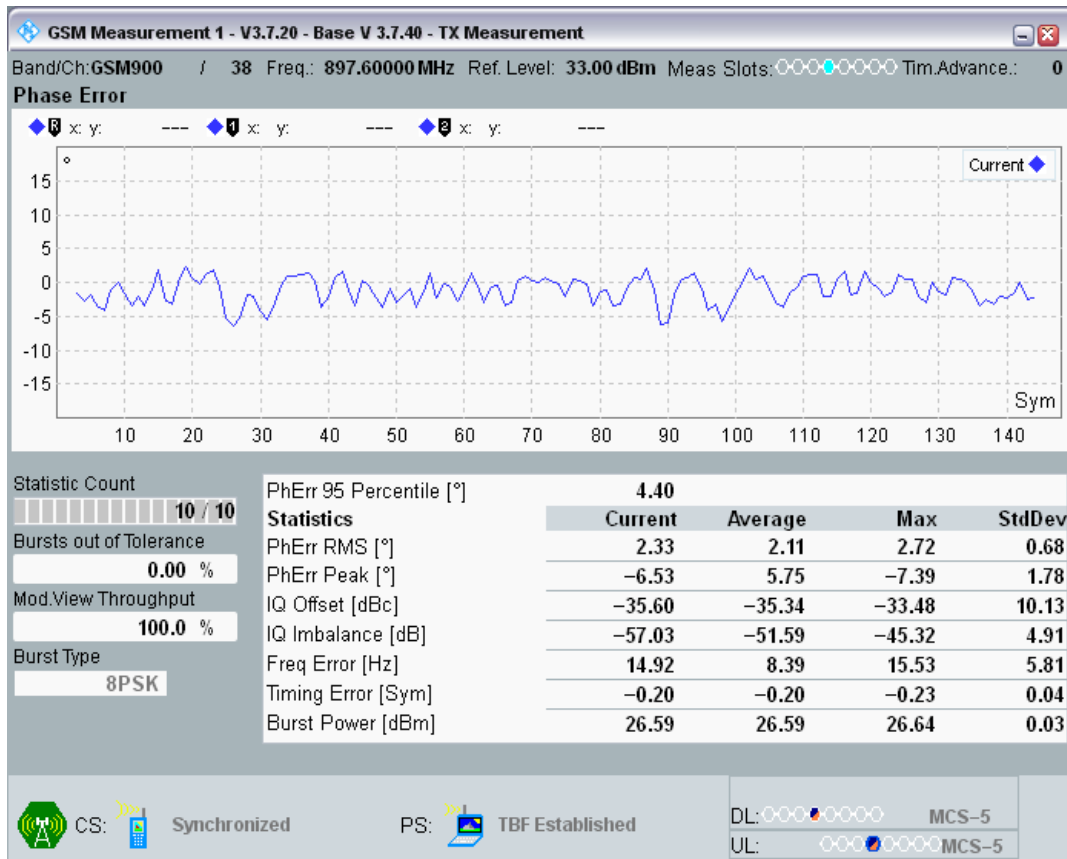
EGPRS900 Channel=38 Gamma=6;6;6;6 HT100 @Sens2
