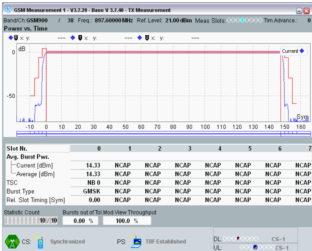
GPRS900 Channel=38 Gamma=11;11;11;11
