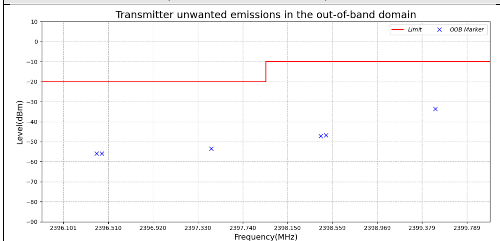
Test_Graph_LE2M_TX_2402_2Mbps_OOB_L
