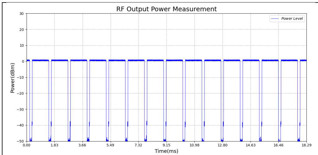
Test_Graph_LE2M_TX_2402_2Mbps_Power_NT
