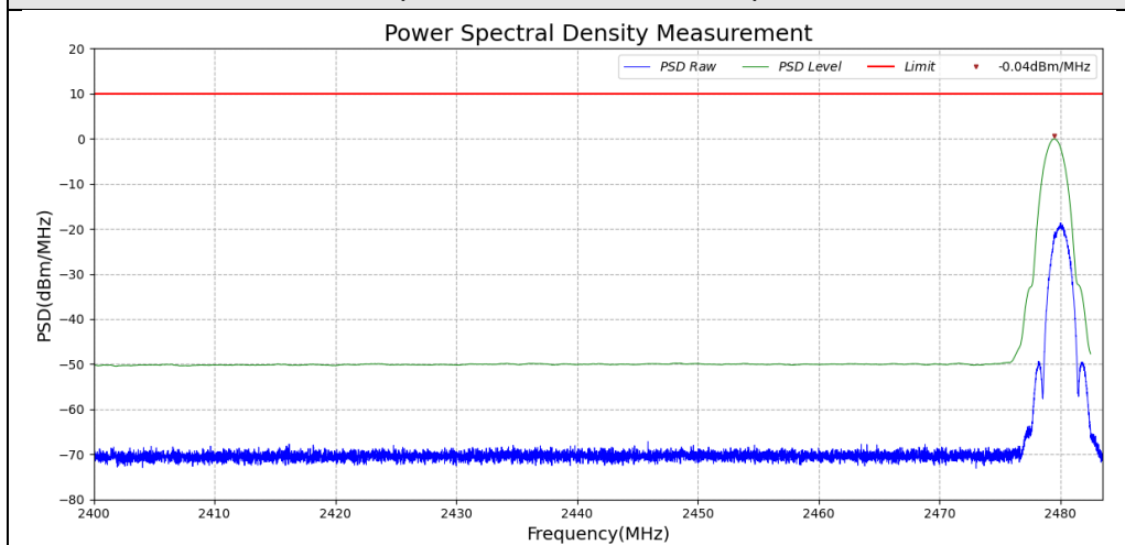
Test_Graph_LE2M_TX_2480_2Mbps_PSD
