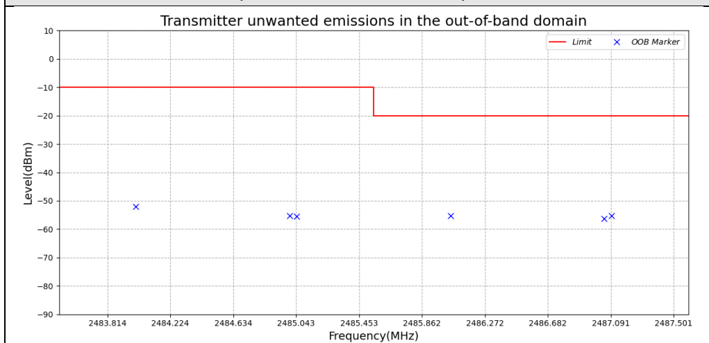
Test_Graph_LE2M_TX_2480_2Mbps_OOB_R
