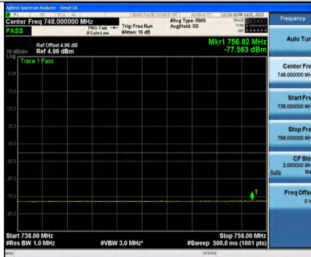
NTNV-Band3-20MHz-QPSK-19575-1RB#0-753~783-1000-3000
