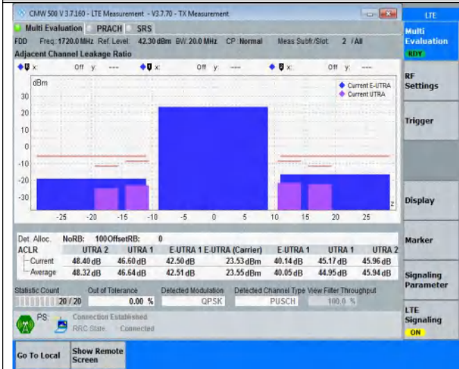
NTNV-Band3-20MHz-QPSK-19575-18RB#82
