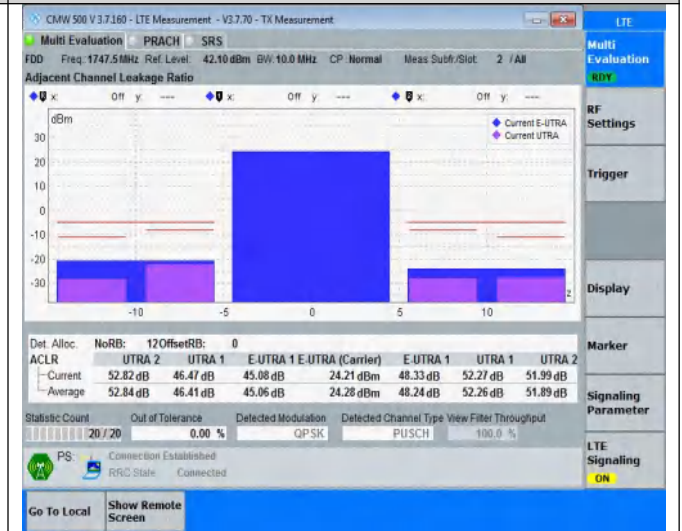
NTNV-Band3-10MHz-QPSK-19575-50RB#0
