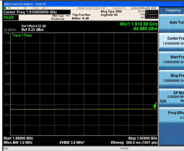
NTNV-Band3-20MHz-QPSK-19575-100RB#0-2110~2170-1000-3000
