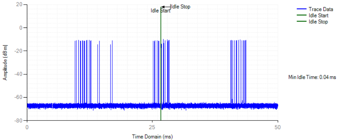
COT NVNT 802.11ac80 5210MHz
