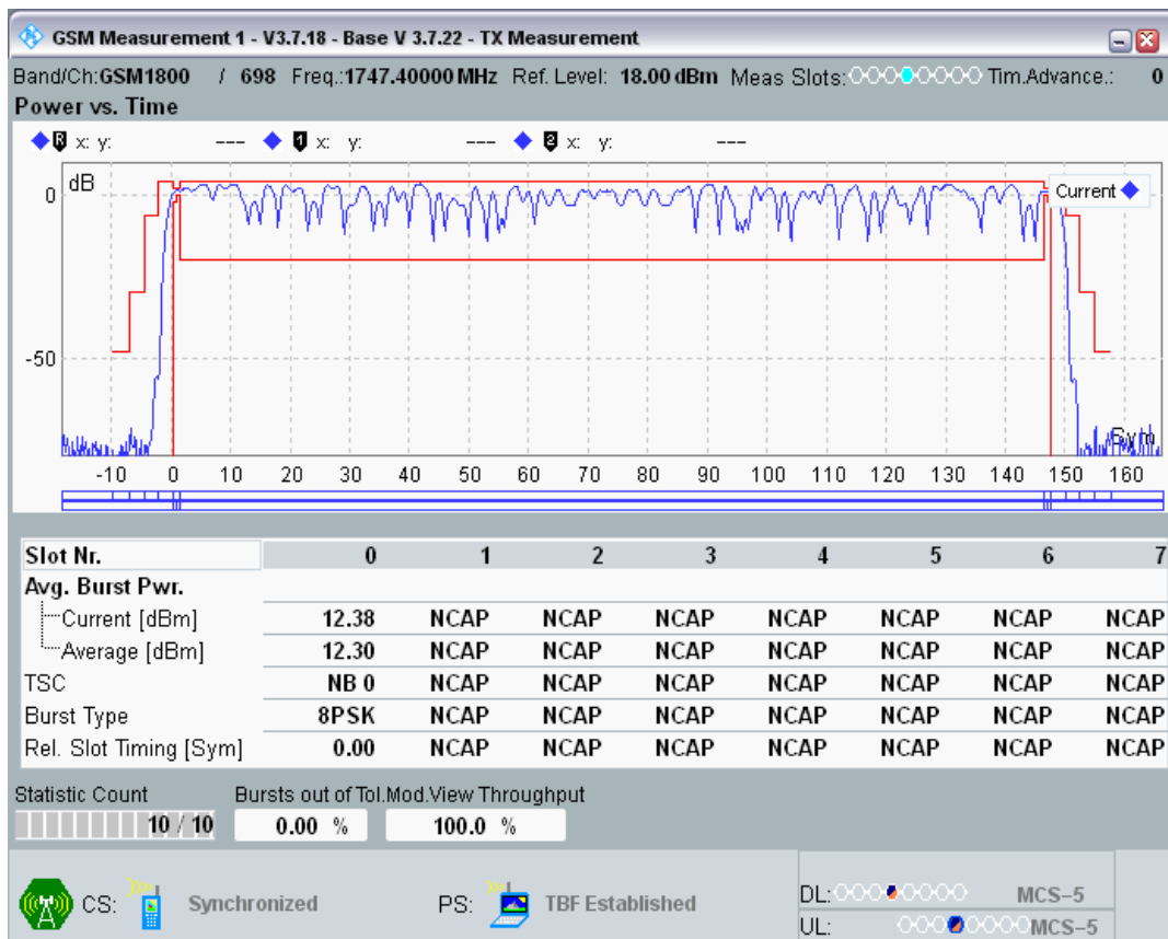
EGPRS1800 Channel=698 Gamma=15;15;15;15
