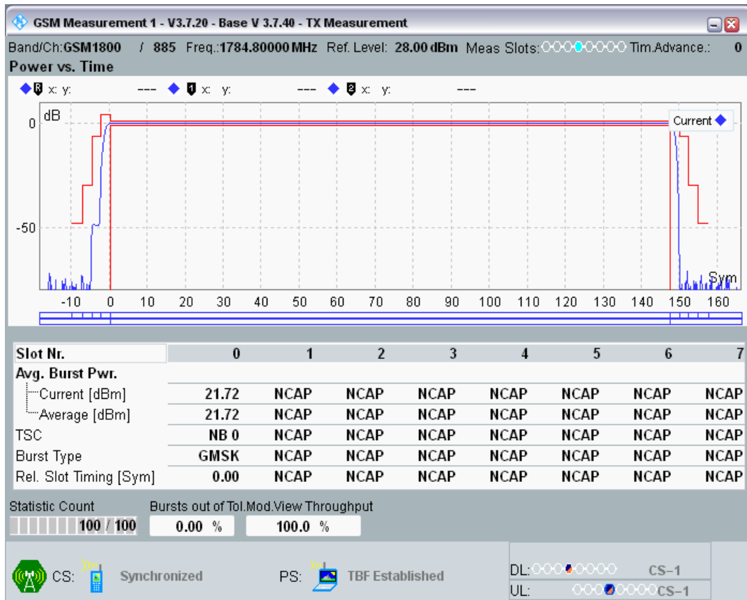
GPRS1800 Channel=885 Gamma=5;5;5;5
