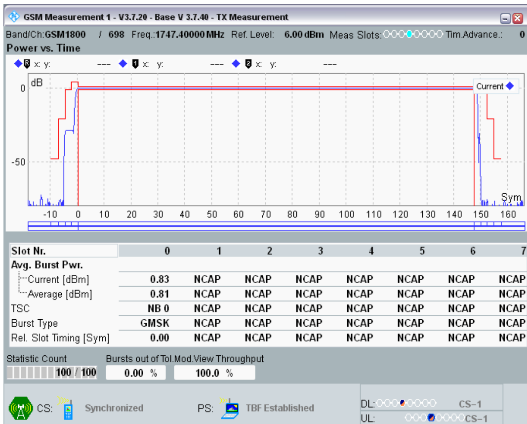
GPRS1800 Channel=512 Gamma=10;10;10;10
