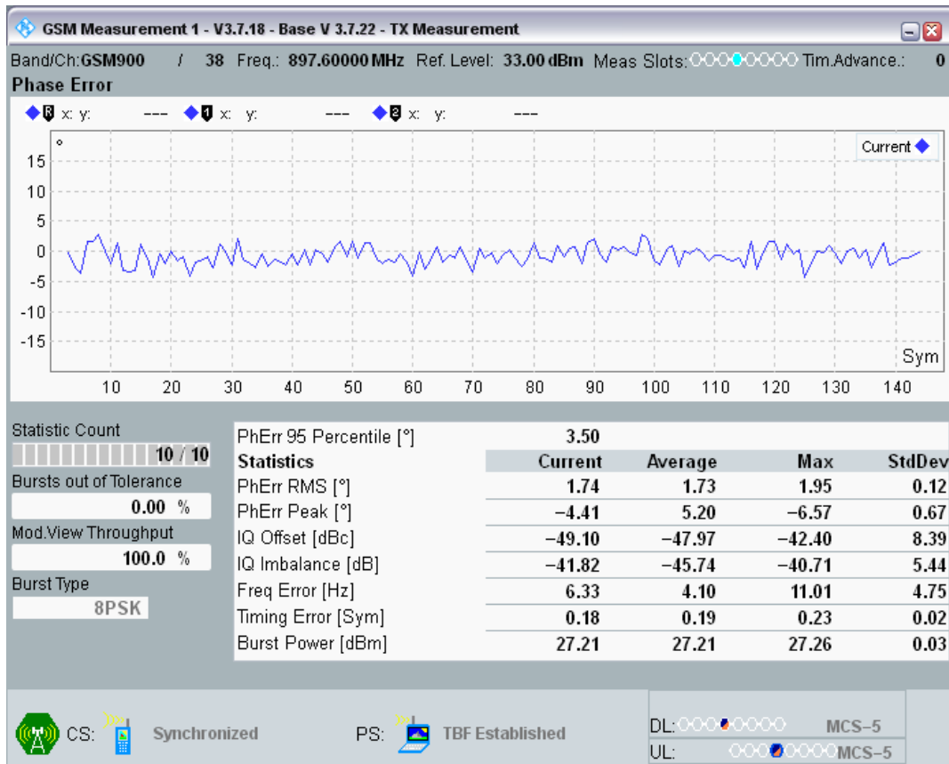
EGPRS900 Channel=38 Gamma=6;6;6;6 TU3 @15
