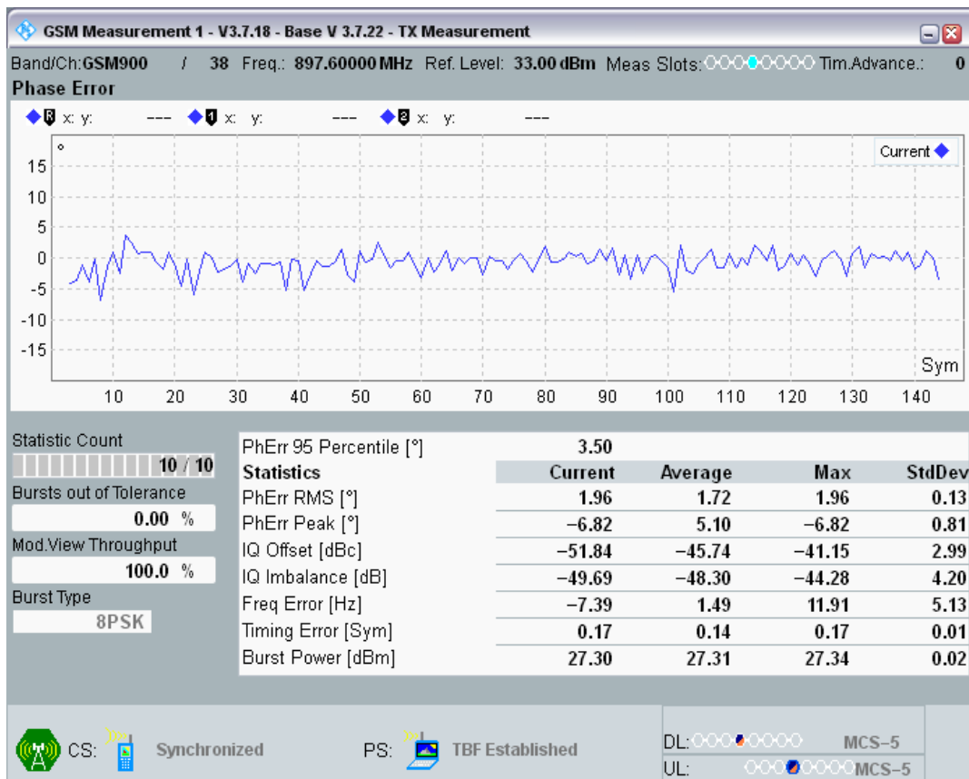
EGPRS900 Channel=38 Gamma=6;6;6;6 TU50 @Sens2
