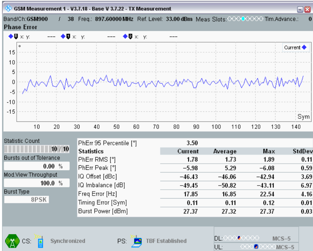
EGPRS900 Channel=38 Gamma=6;6;6;6 TU3 @17
