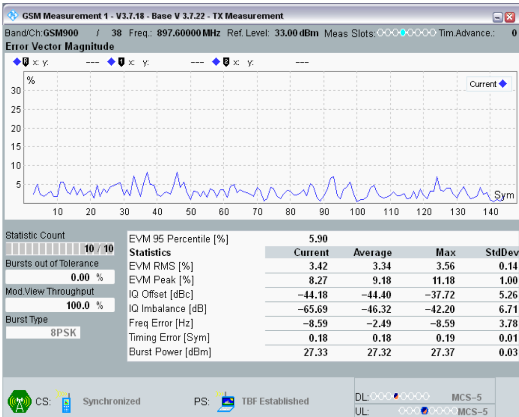
EGPRS900 Channel=38 Gamma=6;6;6;6 RA250 @Sens5
