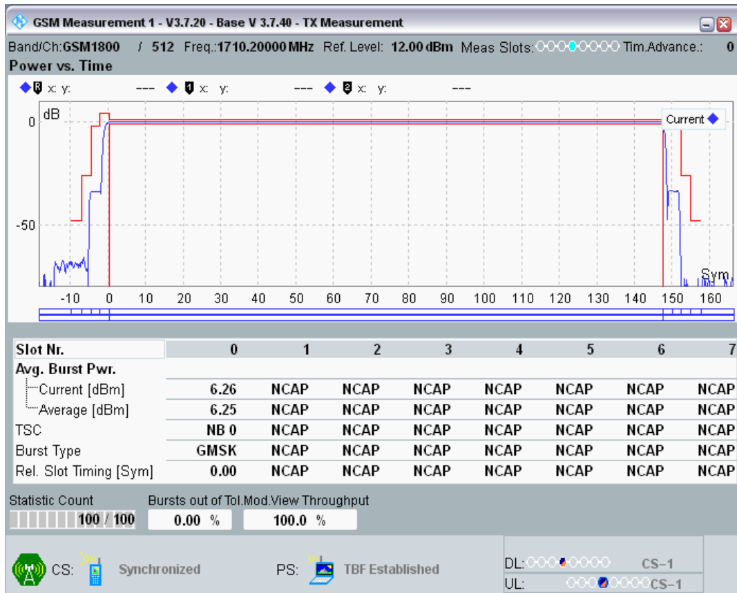
GPRS1800 Channel=512 Gamma=14;14;14;14
