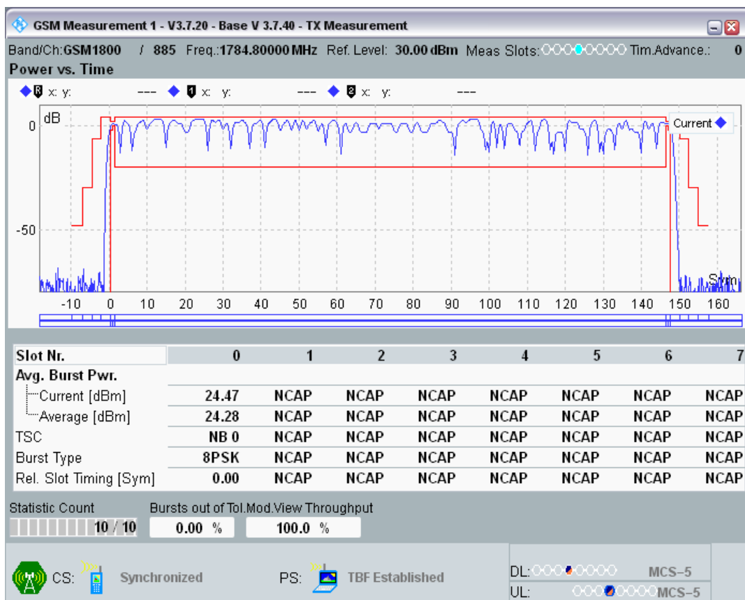
EGPRS1800 Channel=885 Gamma=9;9;9
