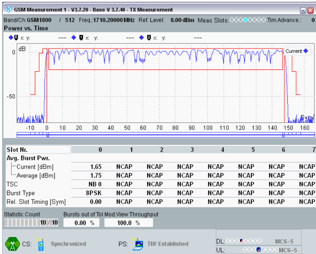
EGPRS1800 Channel=512 Gamma=5;5;5;5
