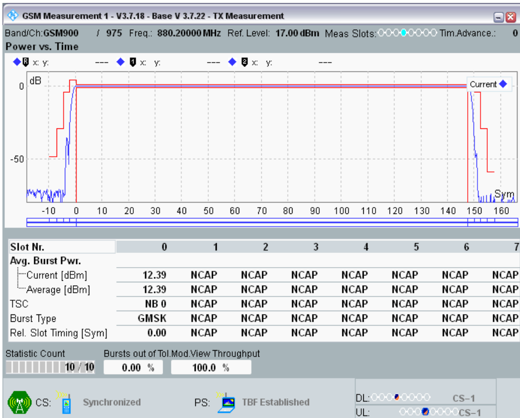
GPRS900 Channel=975 Gamma=15;15;15;15
