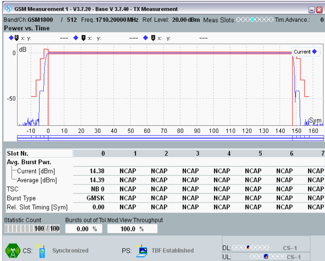
GPRS1800 Channel=512 Gamma=13;13;13;13
