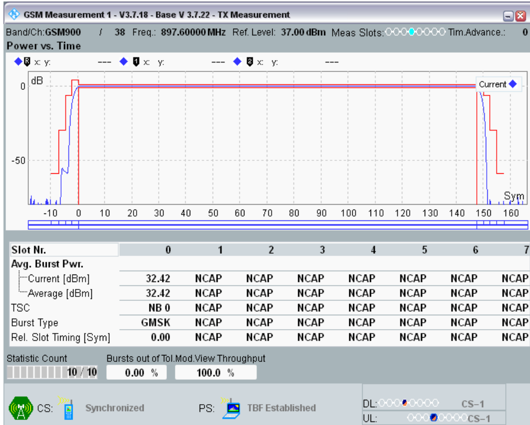
GPRS900 Channel=38 Gamma=5;5;5;5
