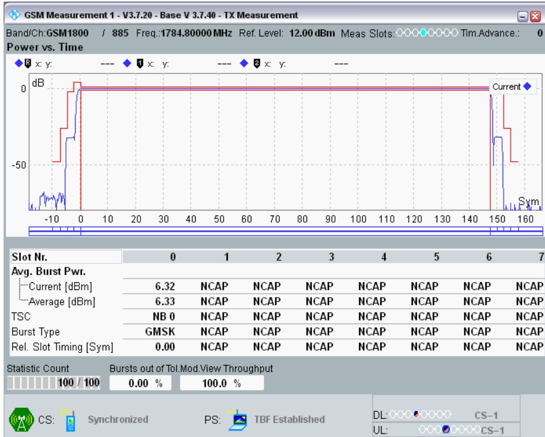
GPRS1800 Channel=885 Gamma=17;17;17;17
