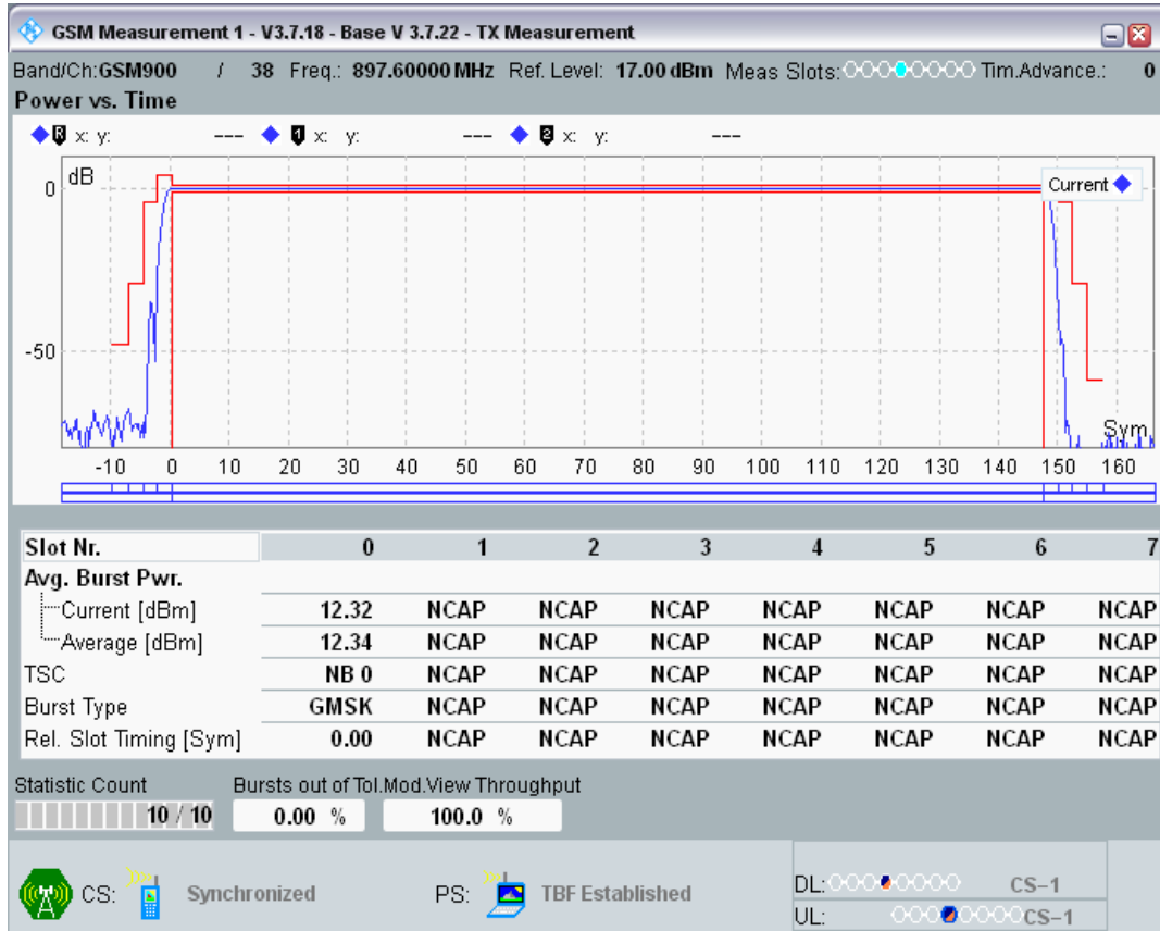
GPRS900 Channel=38 Gamma=15;15;15;15
