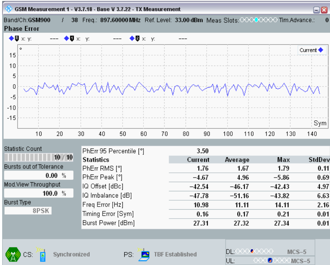
EGPRS900 Channel=38 Gamma=6;6;6;6 TU3 @13
