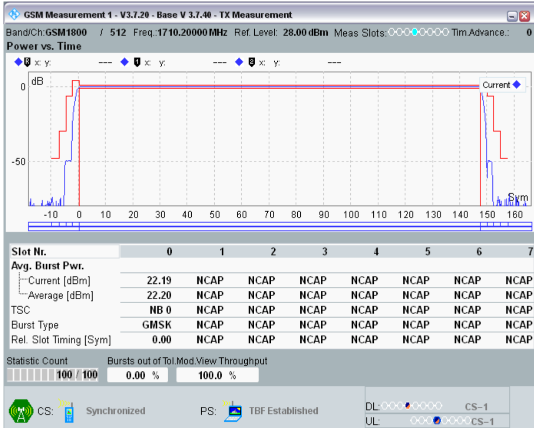
GPRS1800 Channel=512 Gamma=6;6;6;6
