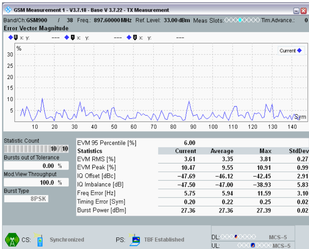
EGPRS900 Channel=38 Gamma=17;17;17;17
