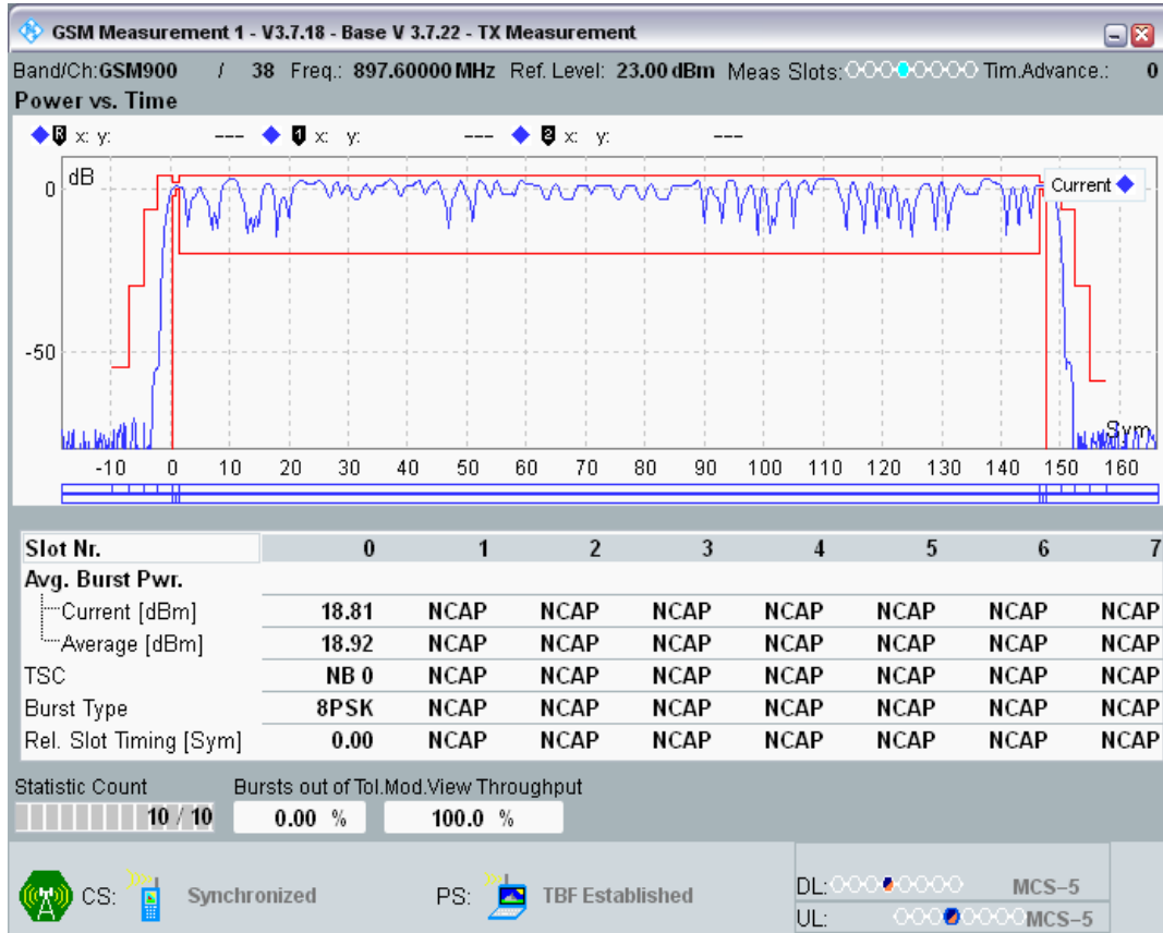
EGPRS900 Channel=38 Gamma=12;12;12;12
