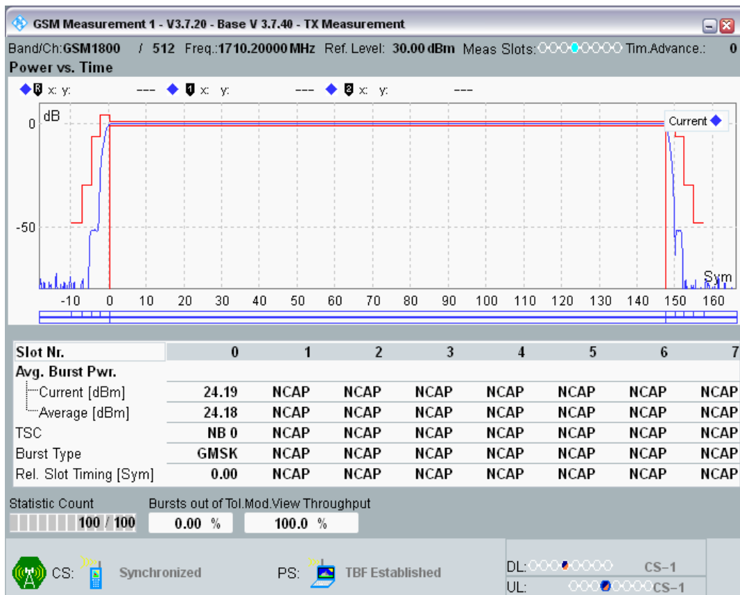
GPRS1800 Channel=512 Gamma=8;8;8;8
