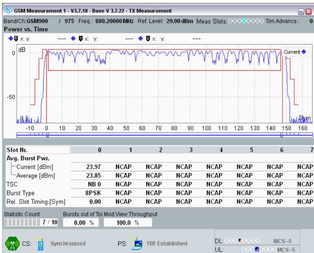
EGPRS900 Channel=975 Gamma=9;9;9;9
