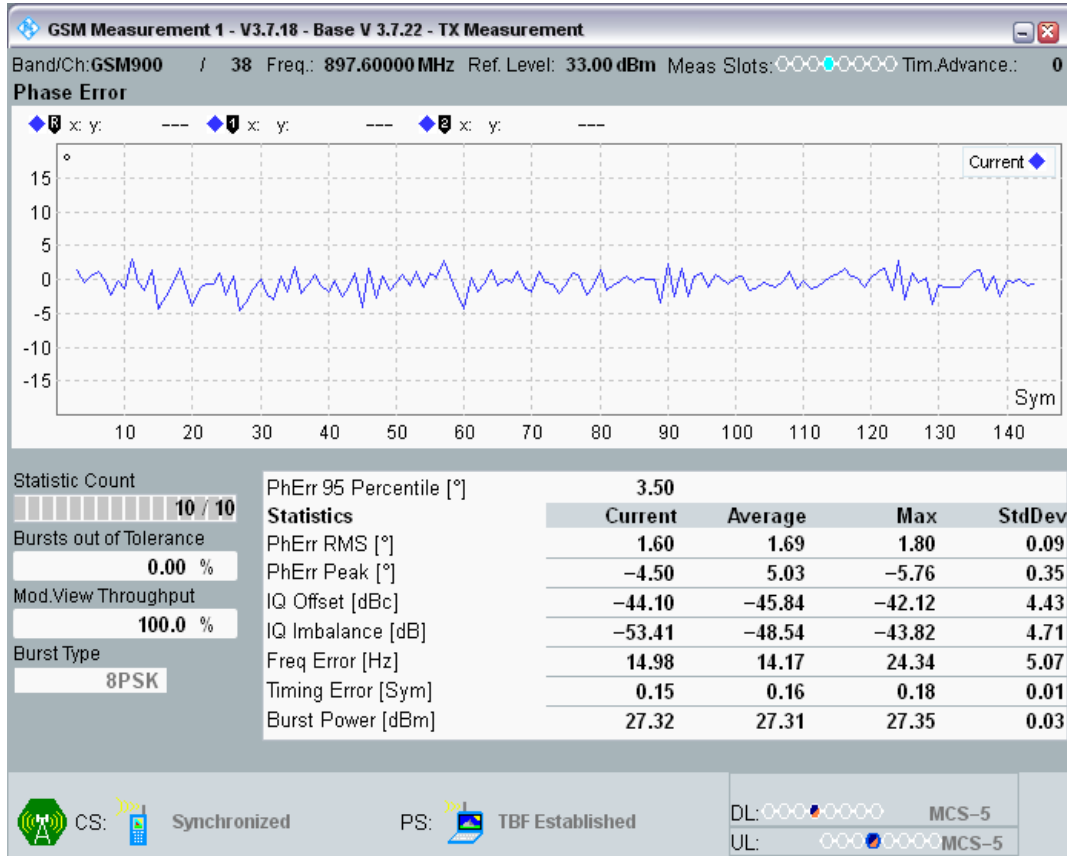
EGPRS900 Channel=38 Gamma=6;6;6;6 HT100 @Sens2
