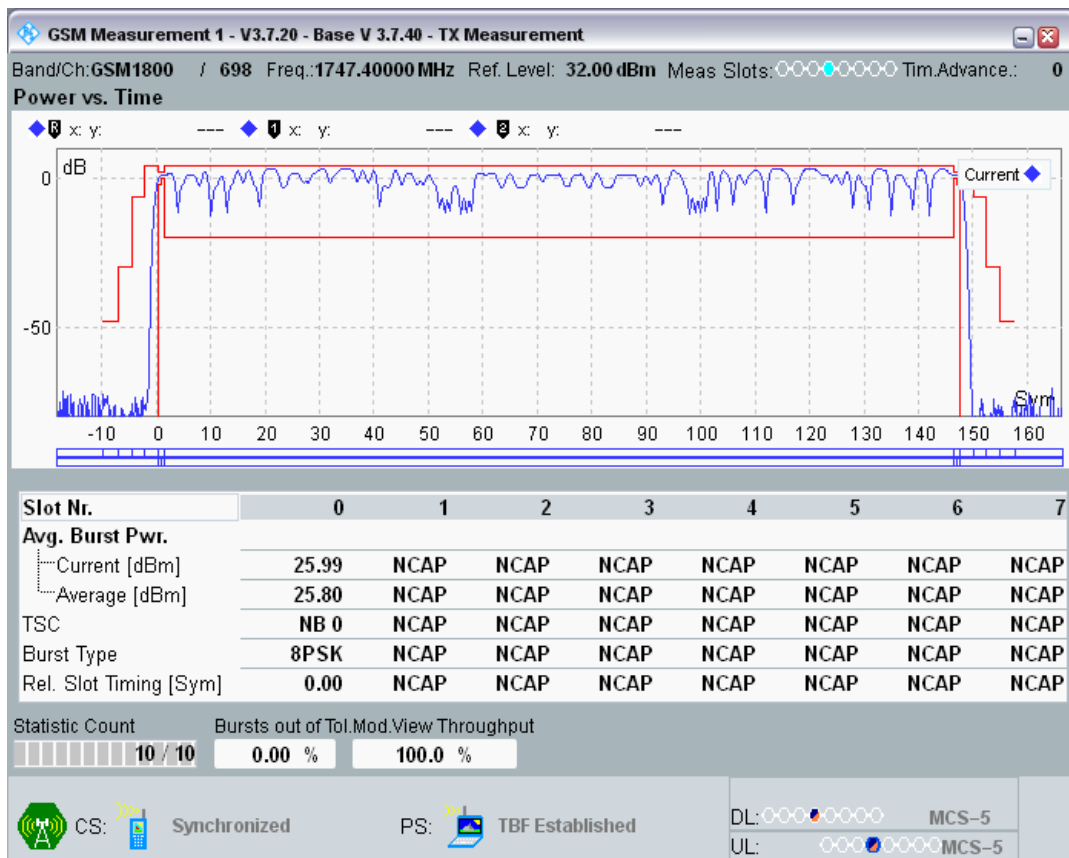
EGPRS1800 Channel=698 Gamma=6;6;6;6
