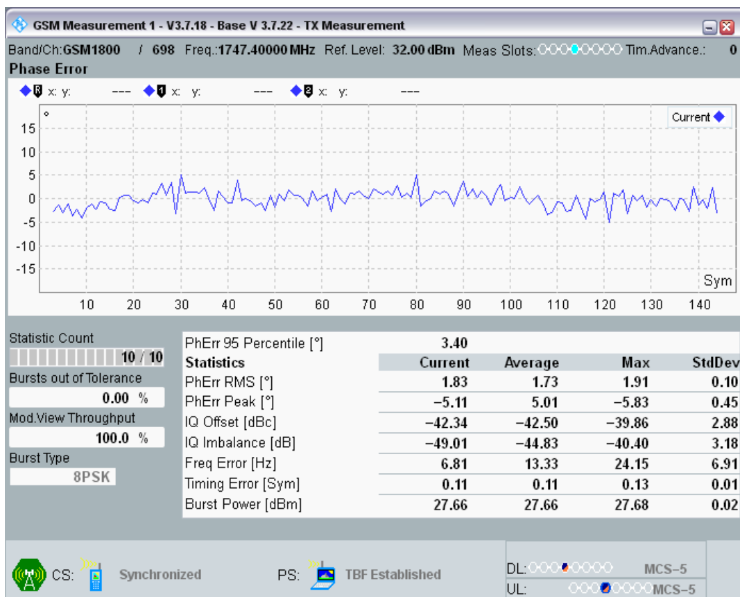
EGPRS1800 Channel=698 Gamma=5;5;5;5 TU3 @10
