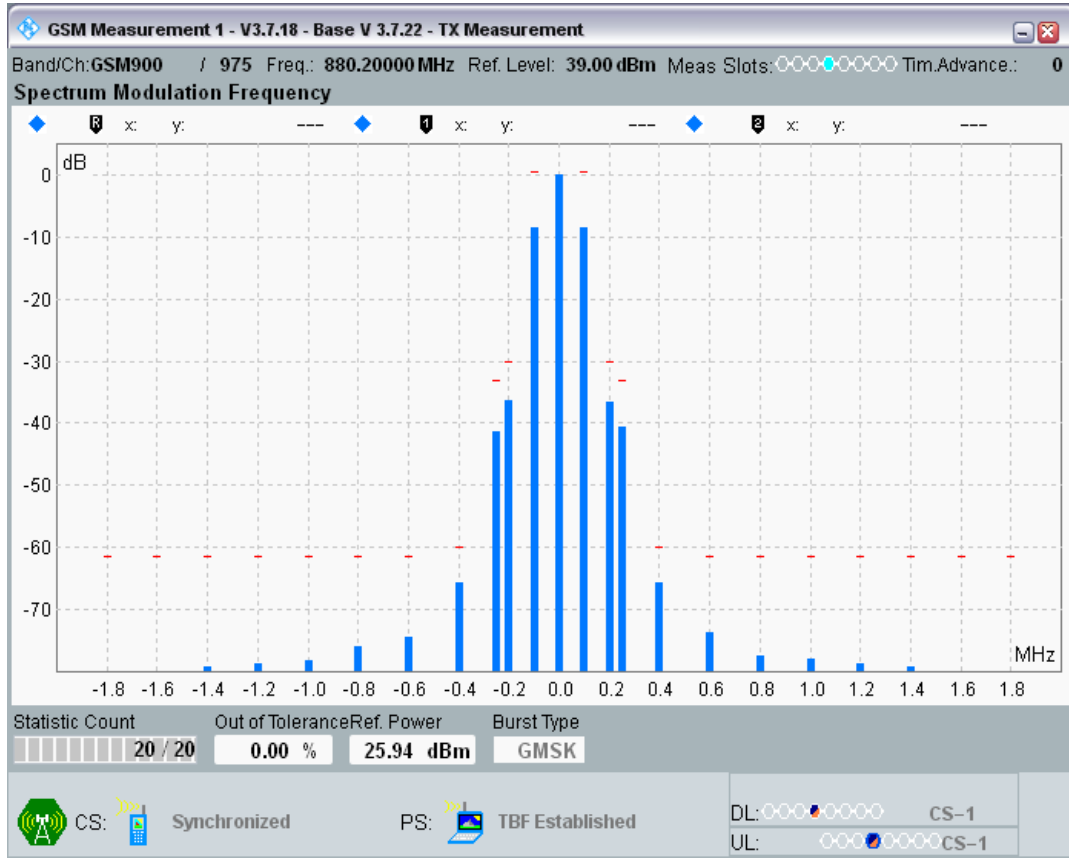
GPRS900 Channel=975 Gamma=17;17;17;17
