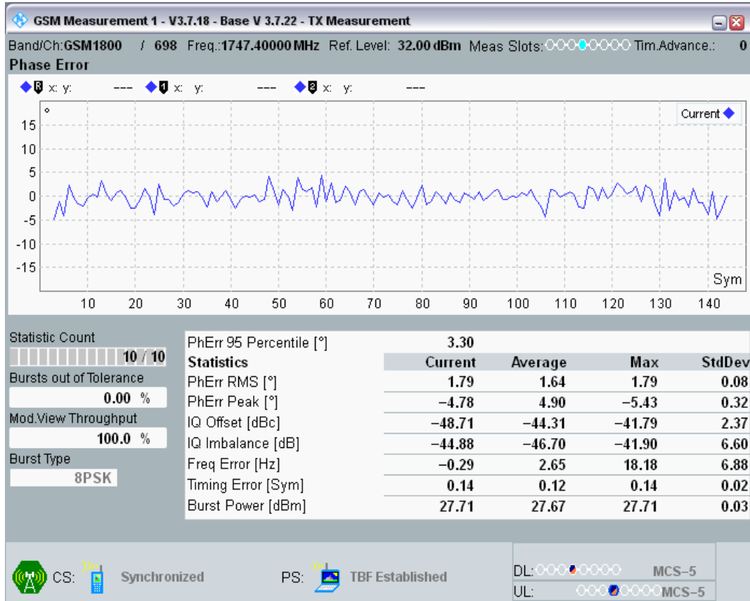
EGPRS1800 Channel=698 Gamma=5;5;5;5 TU3 @9
