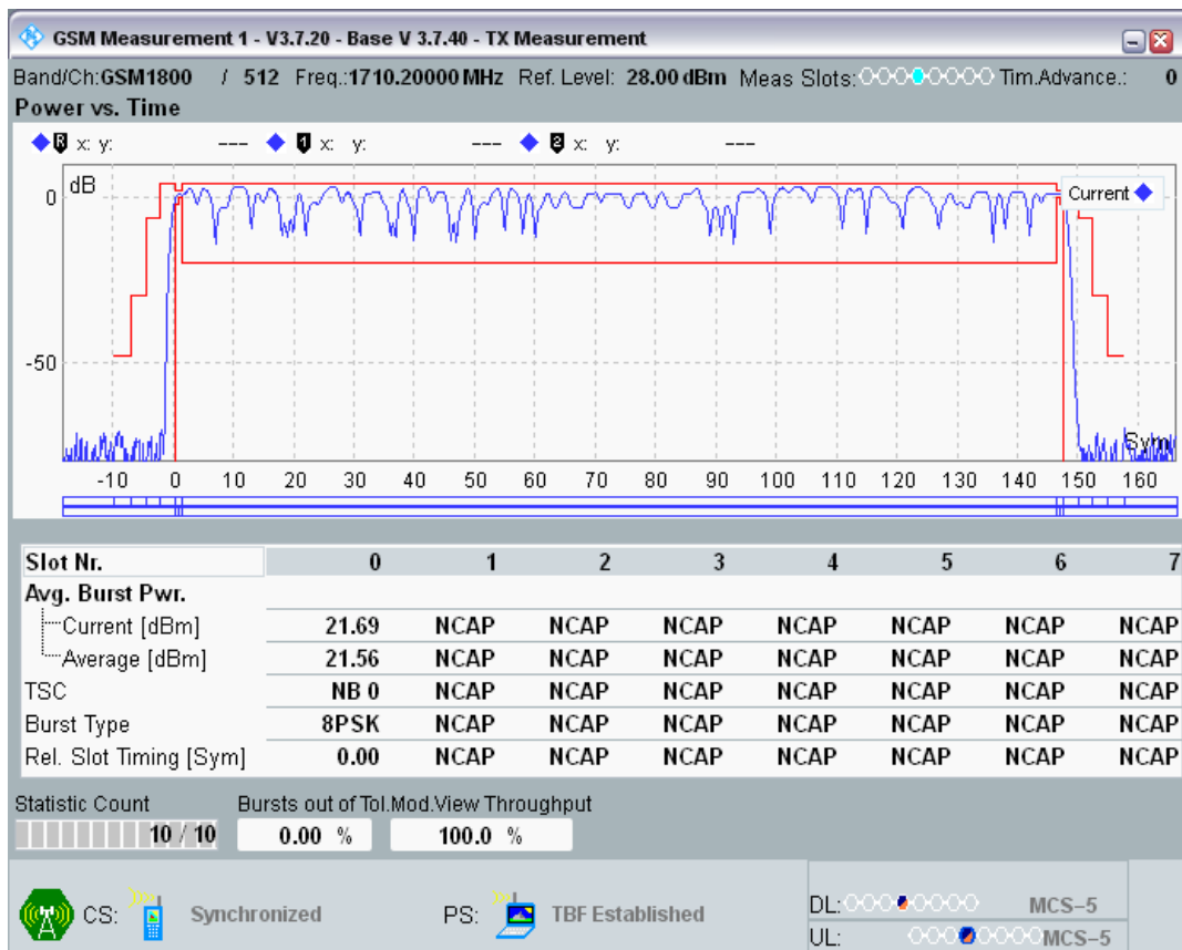
EGPRS1800 Channel=698 Gamma=12;12;12;12
