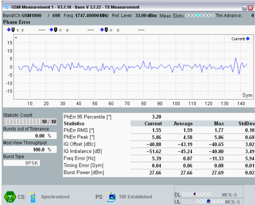
EGPRS1800 Channel=698 Gamma=5;5;5;5 TU3 @20
