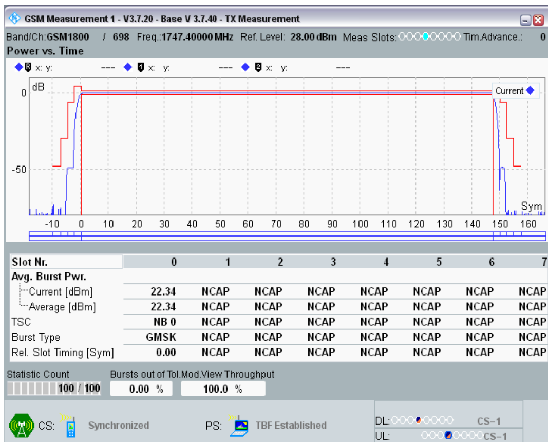
GPRS1800 Channel=885 Gamma=12;12;12;12
