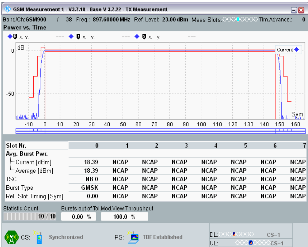
GPRS900 Channel=38 Gamma=12;12;12;12
