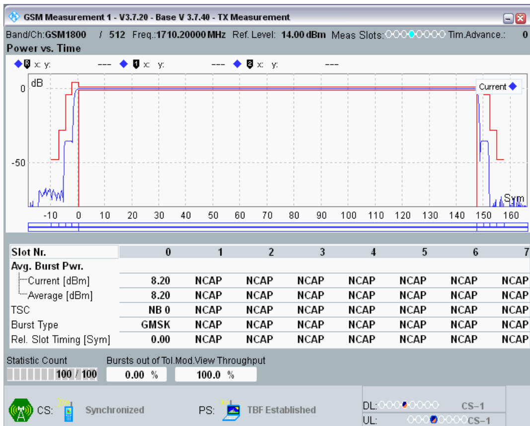
GPRS1800 Channel=698 Gamma=13;13;13;13
