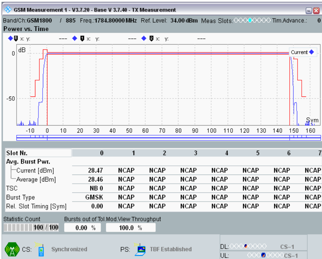
GPRS1800 Channel=885 Gamma=6;6;6;6
