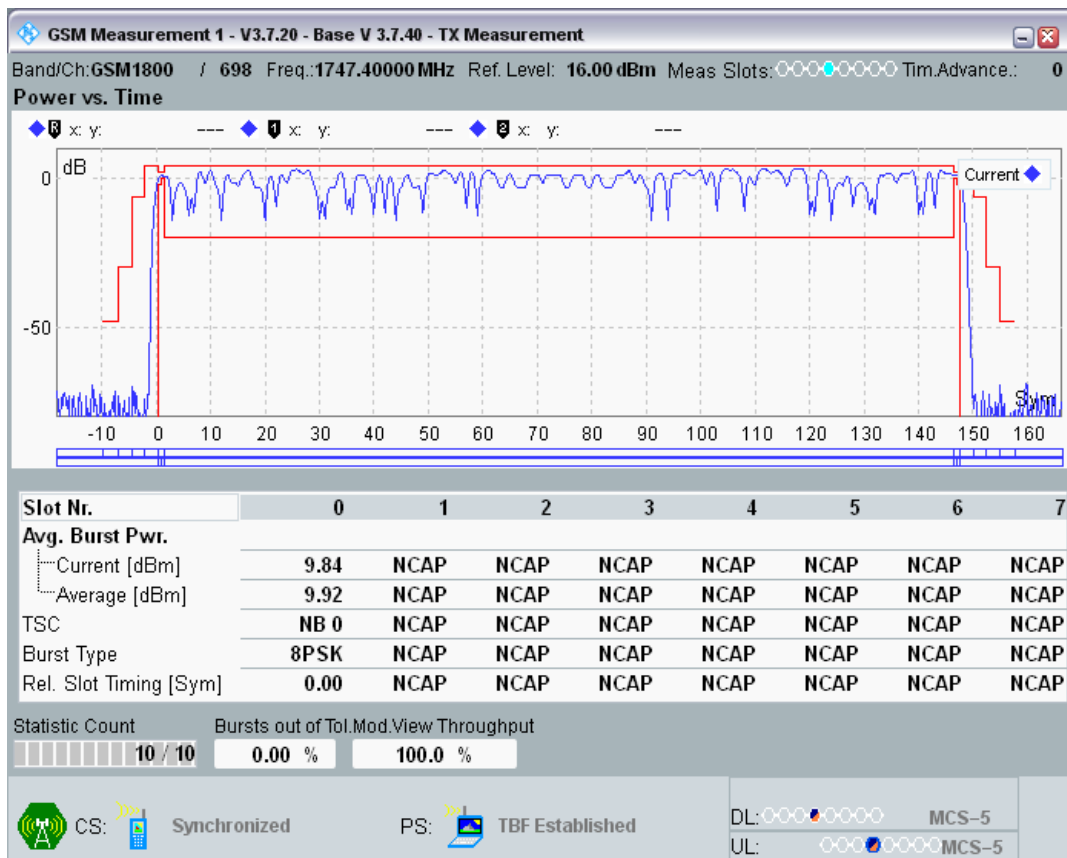
EGPRS1800 Channel=698 Gamma=10;10;10;10
