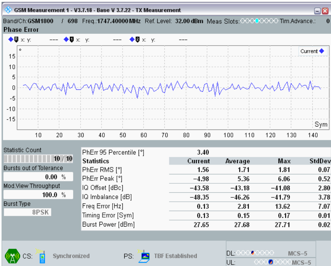
EGPRS1800 Channel=698 Gamma=5;5;5;5 TU50 @Sens5
