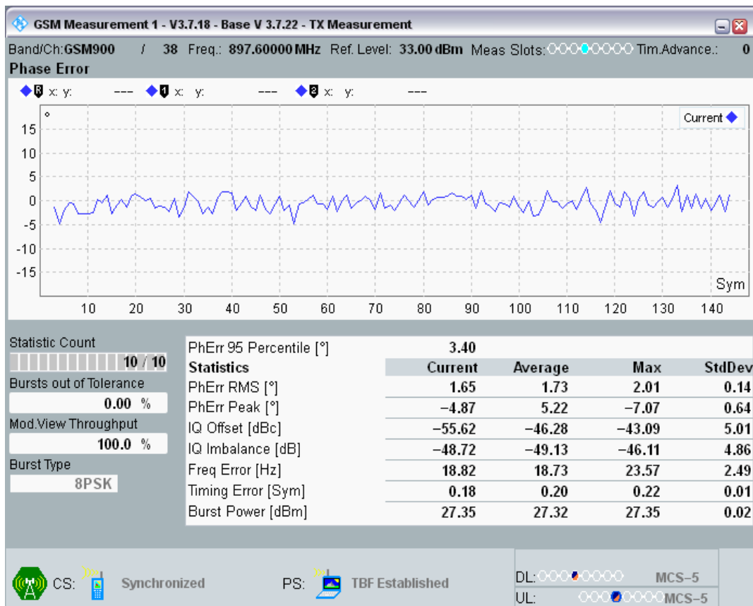
EGPRS900 Channel=38 Gamma=6;6;6;6 RA250 @Sens4
