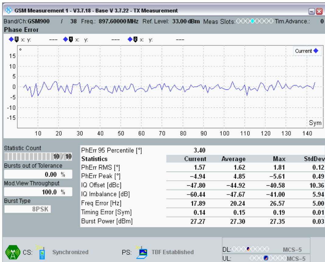
EGPRS900 Channel=38 Gamma=6;6;6;6 TU3 @14
