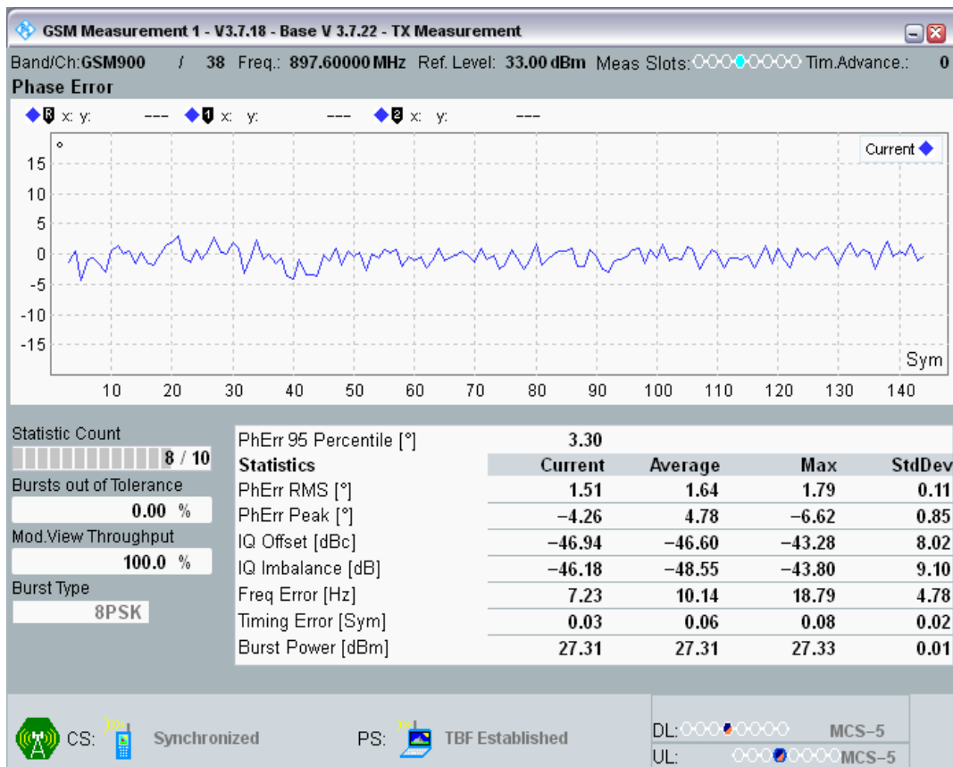
EGPRS900 Channel=38 Gamma=6;6;6;6 TU3 @20
