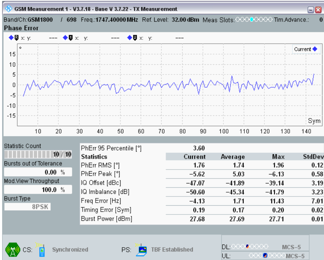
EGPRS1800 Channel=698 Gamma=5;5;5;5 HT100 @Sens2
