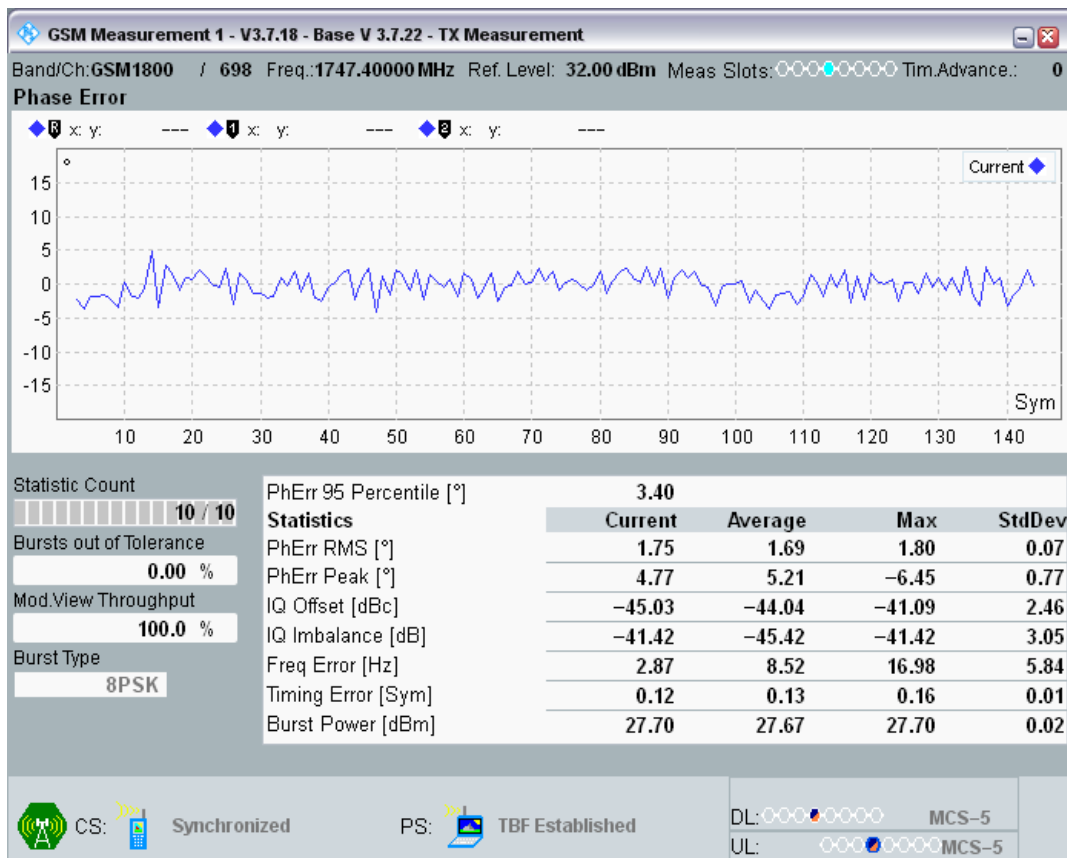
EGPRS1800 Channel=698 Gamma=5;5;5;5 TU3 @6
