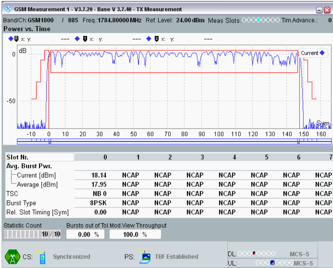
EGPRS1800 Channel=885 Gamma=8;8;8;8
