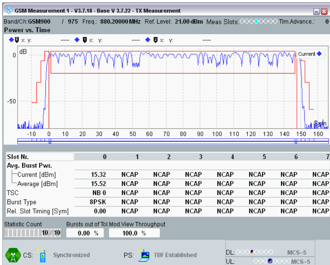
EGPRS900 Channel=975 Gamma=13;13;13;13
