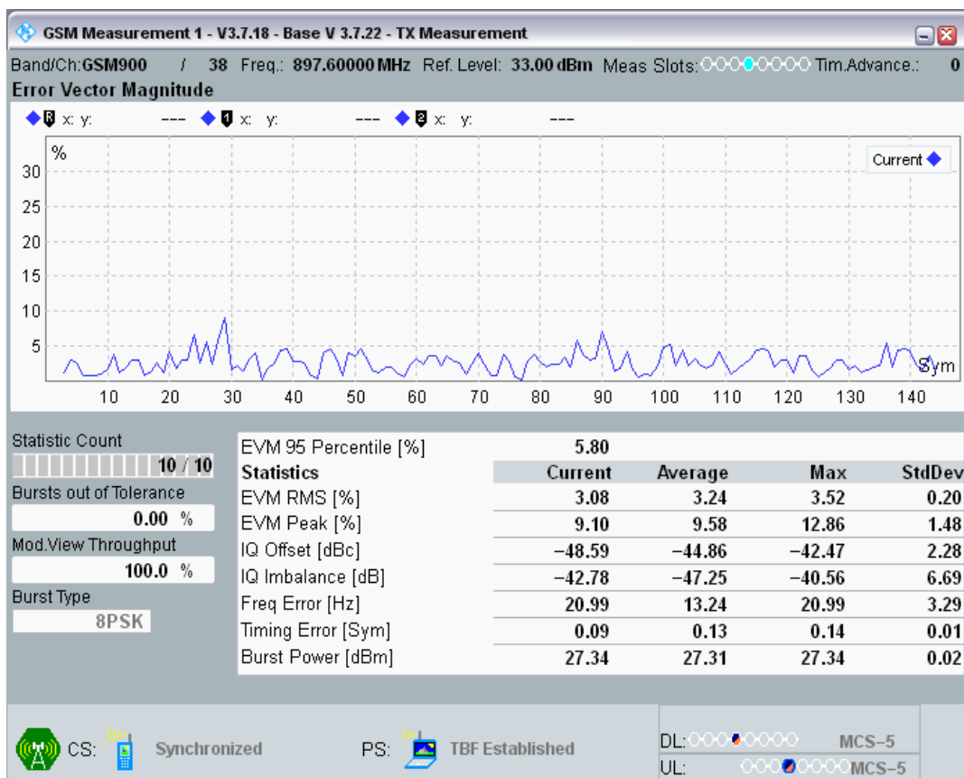
EGPRS900 Channel=38 Gamma=6;6;6;6 TU3 @2
