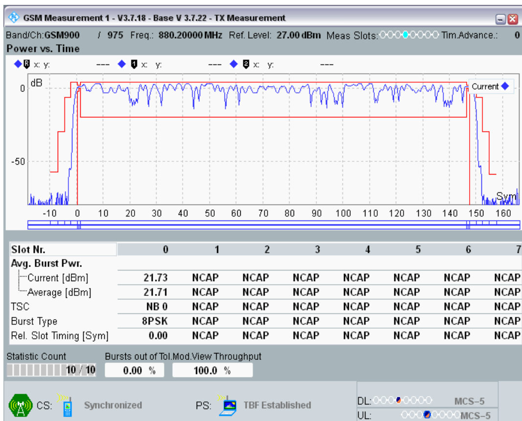
EGPRS900 Channel=975 Gamma=10;10;10;10
