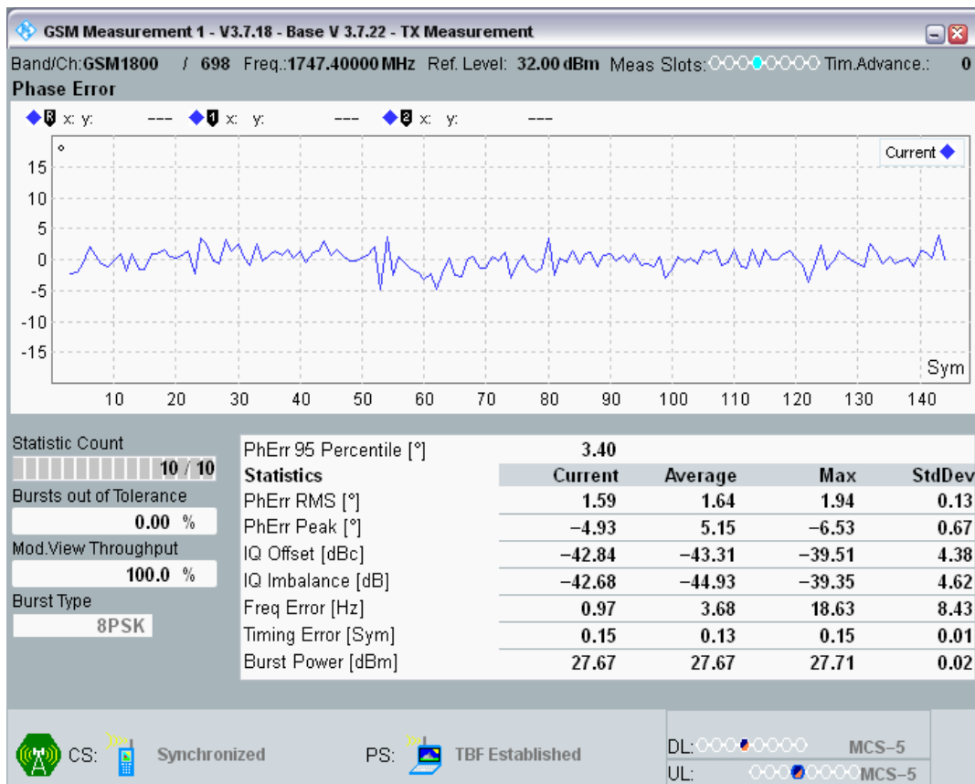
EGPRS1800 Channel=698 Gamma=5;5;5;5 TU3 @7
