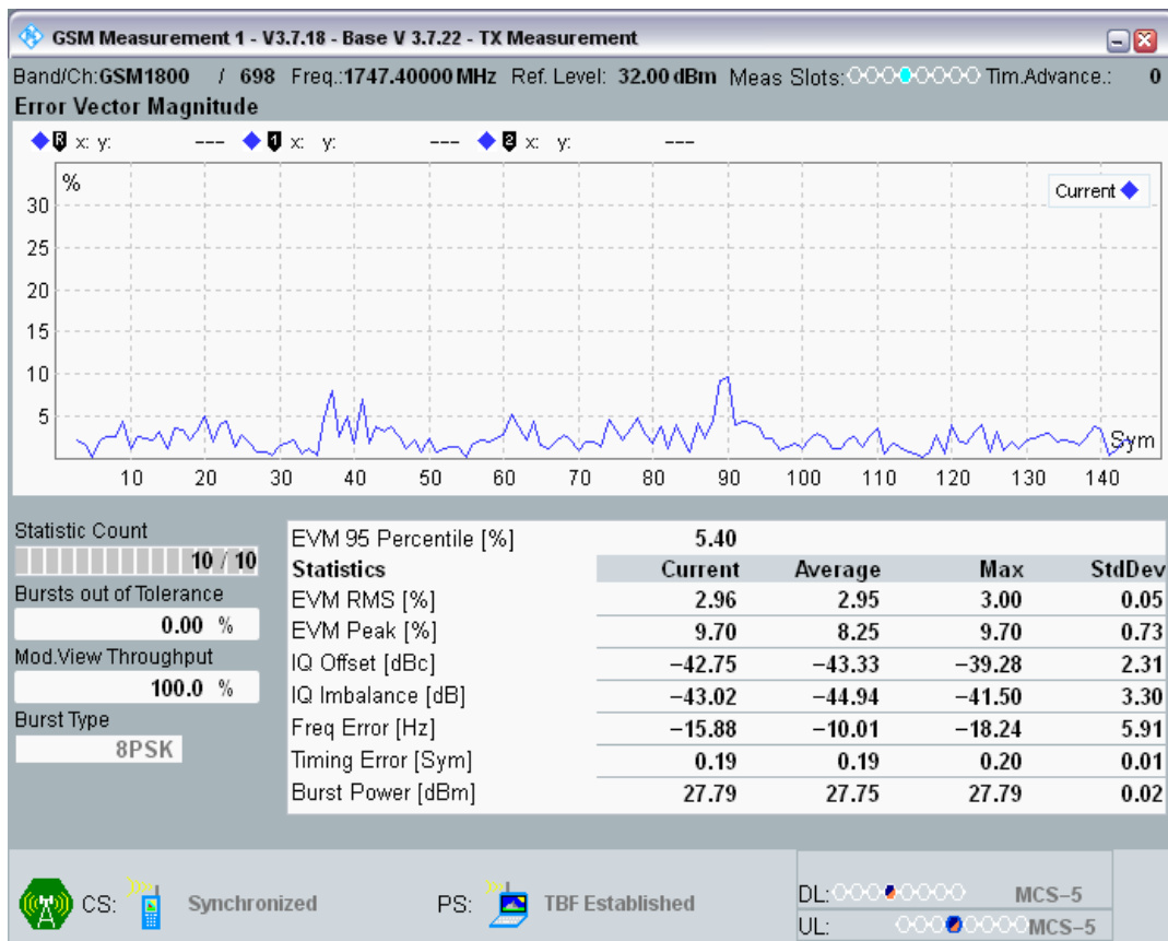
EGPRS1800 Channel=698 Gamma=18;18;18;18
