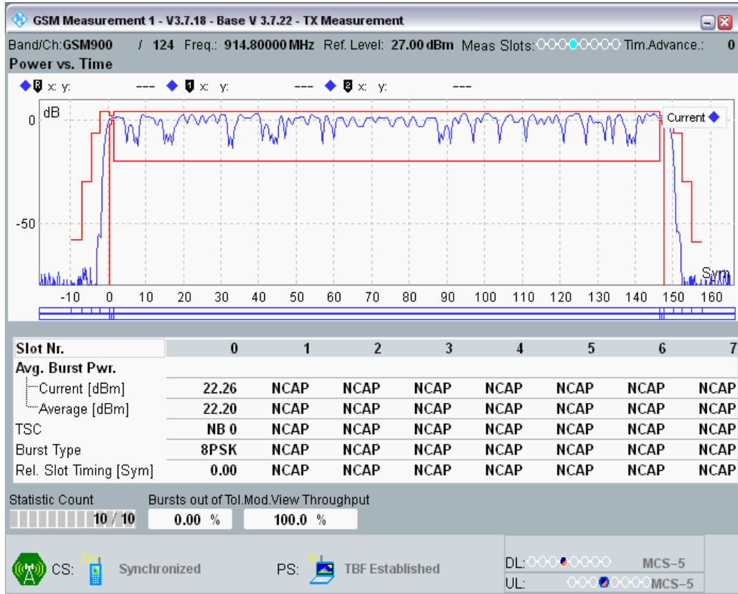
EGPRS900 Channel=124 Gamma=10;10;10;10
