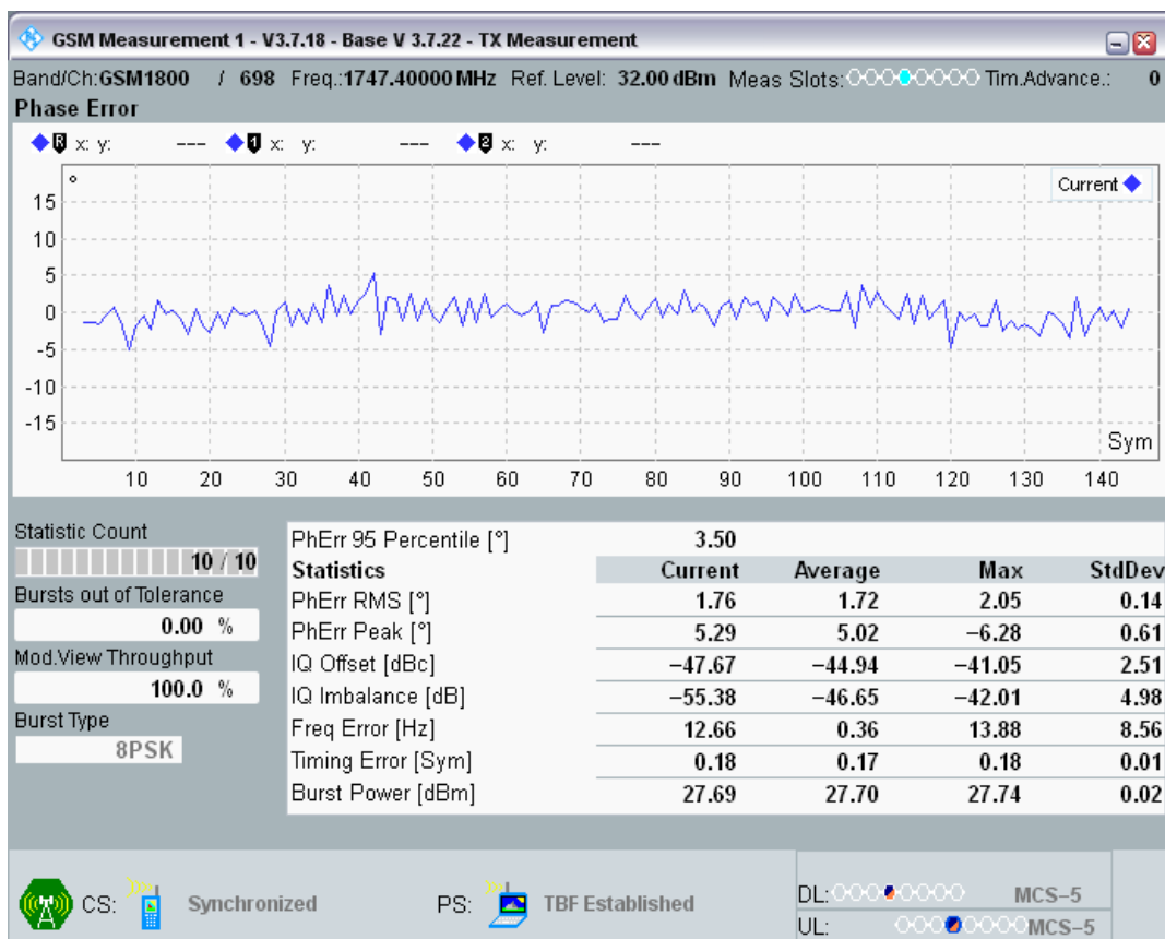
EGPRS1800 Channel=698 Gamma=5;5;5;5 HT100 @Sens5
