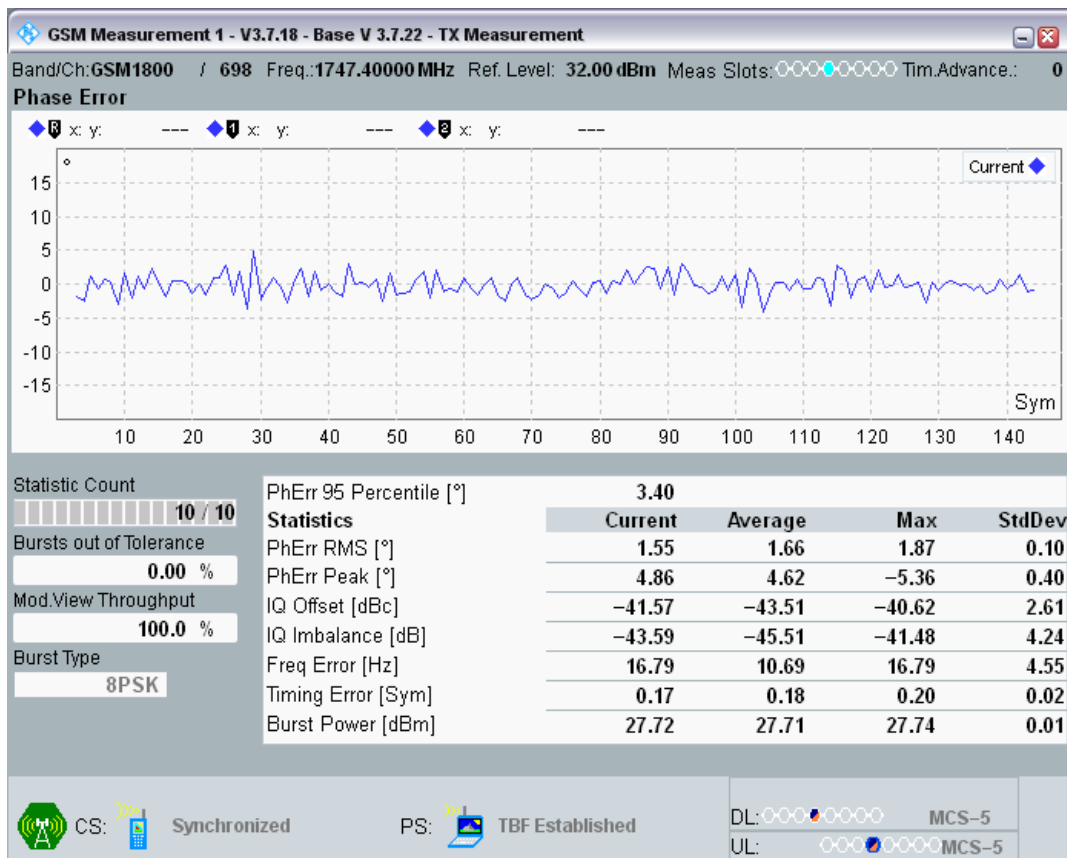
EGPRS1800 Channel=698 Gamma=5;5;5;5 RA250 @Sens3
