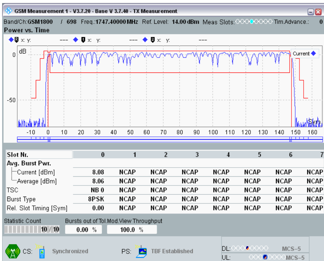
EGPRS1800 Channel=512 Gamma=8;8;8;8
