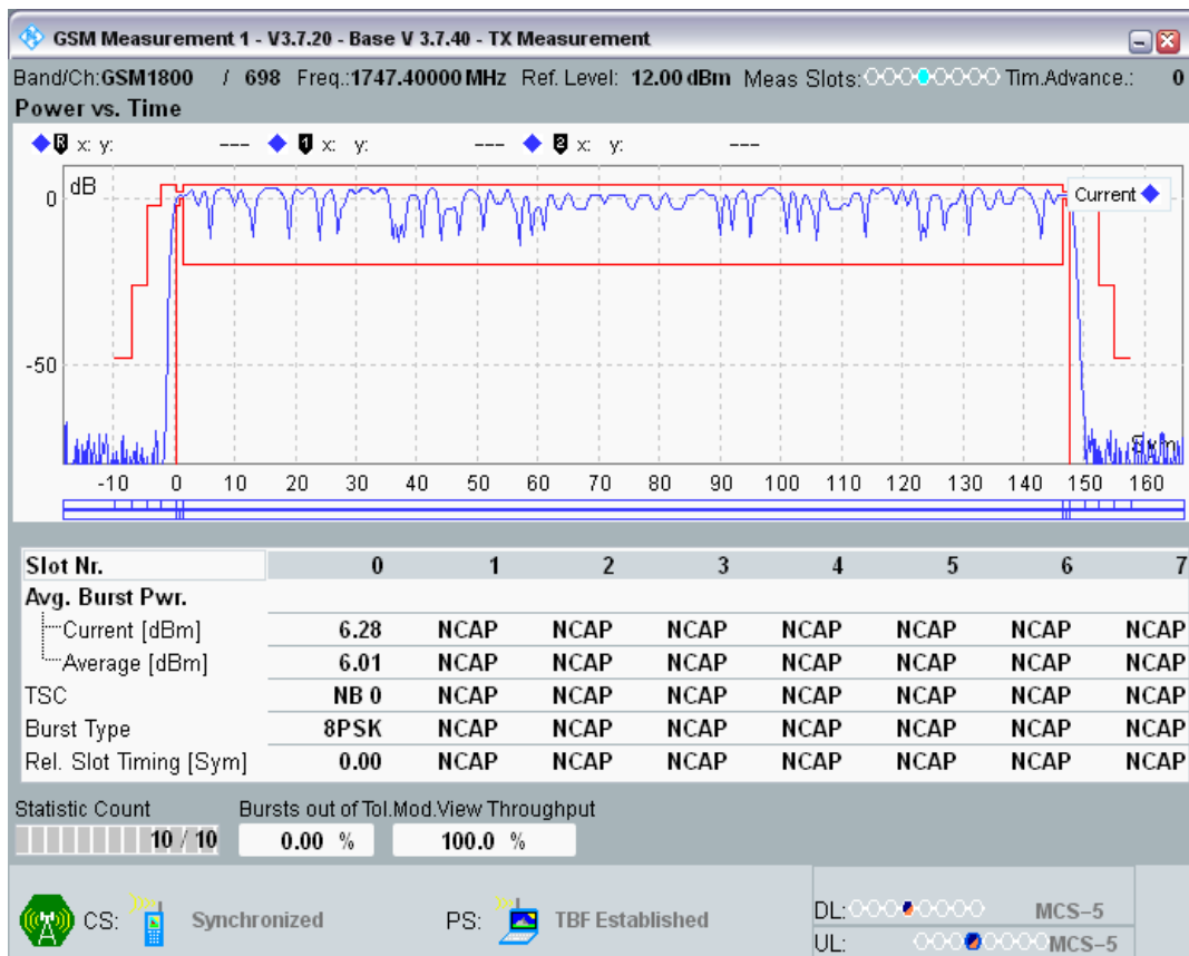
EGPRS1800 Channel=698 Gamma=16;16;16;16
