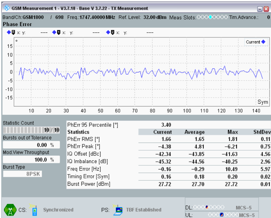
EGPRS1800 Channel=698 Gamma=5;5;5;5 RA250 @Sens5
