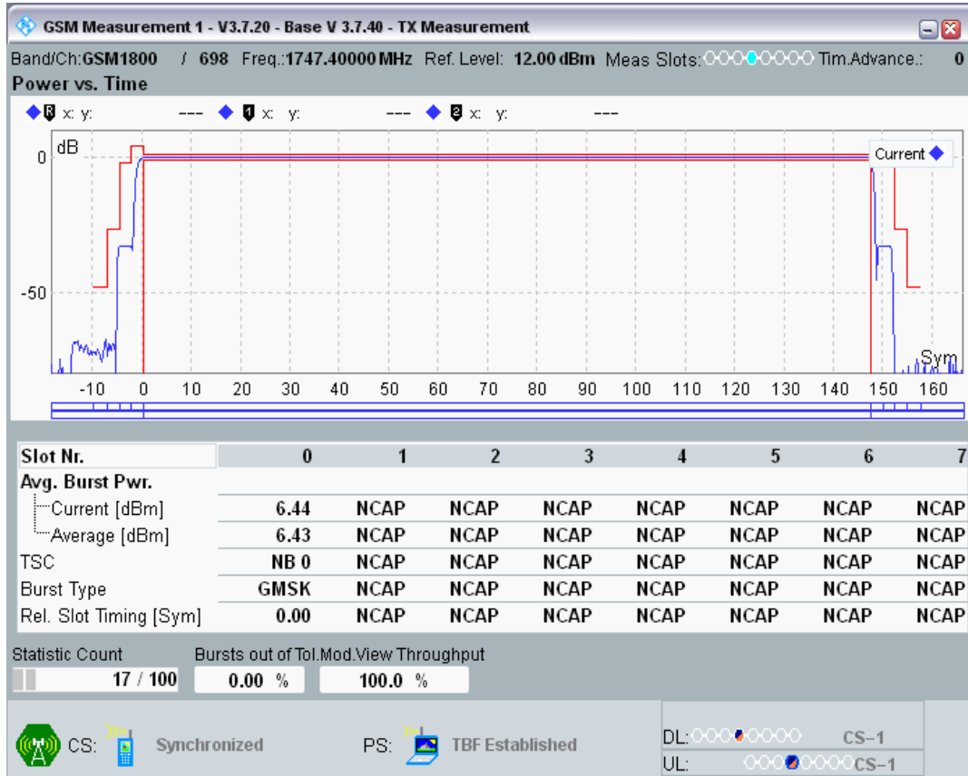
GPRS1800 Channel=698 Gamma=11;11;11;11
