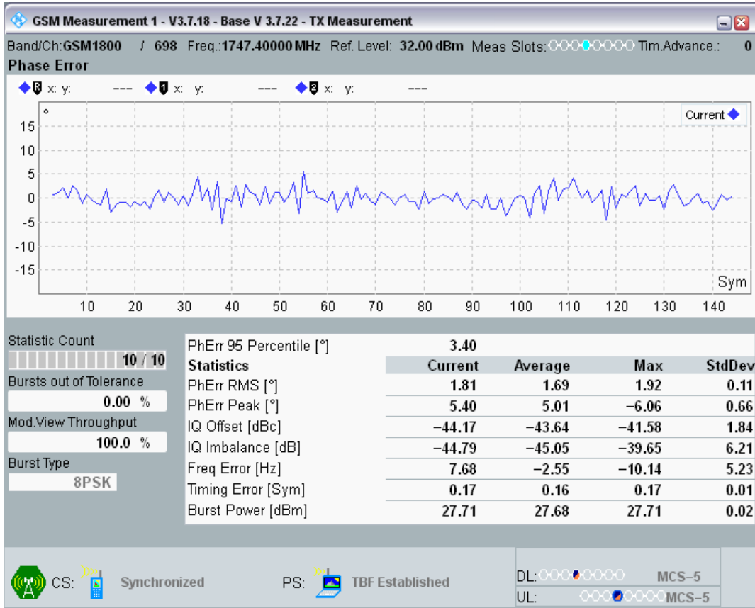
EGPRS1800 Channel=698 Gamma=5;5;5;5 TU50 @Sens4
