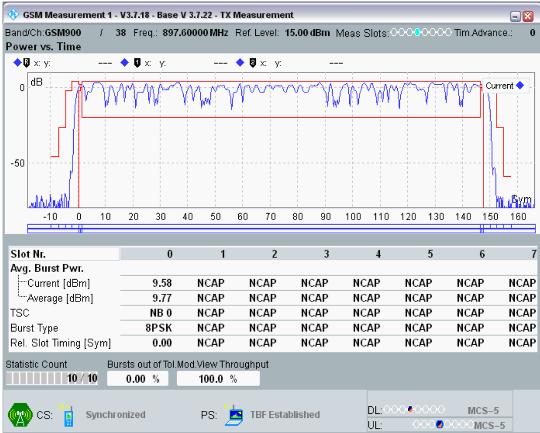
EGPRS900 Channel=38 Gamma=16;16;16;16
