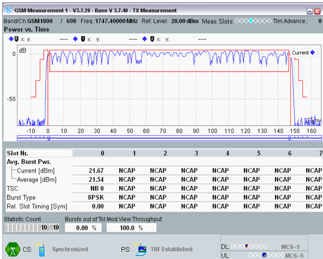
EGPRS1800 Channel=698 Gamma=8;8;8;8
