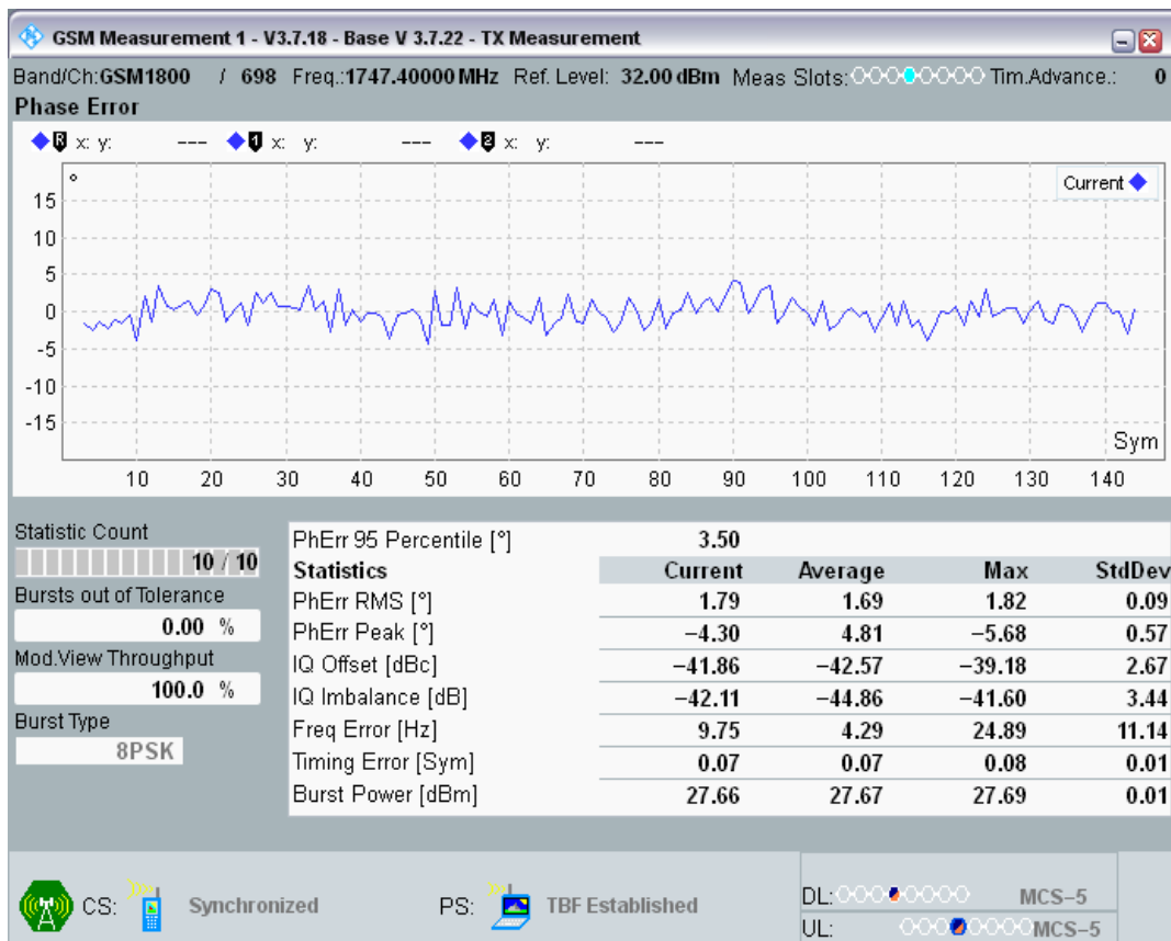
EGPRS1800 Channel=698 Gamma=5;5;5;5 TU3 @19
