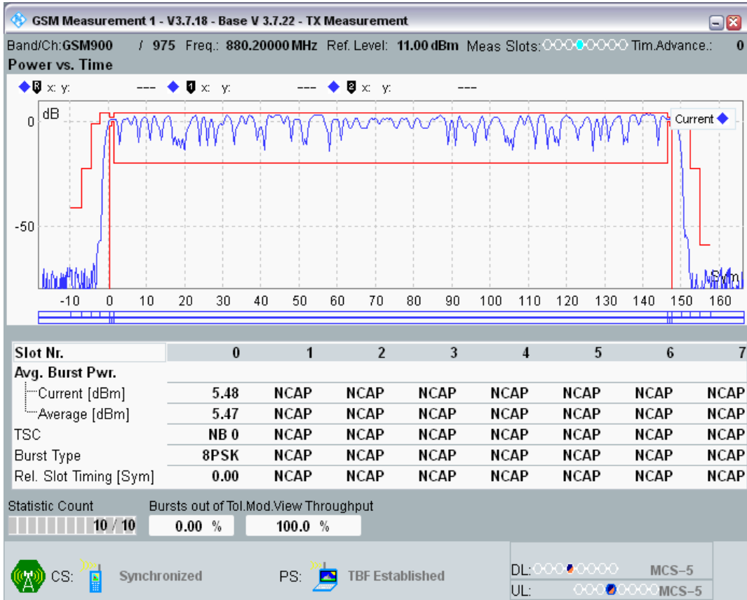
EGPRS900 Channel=38 Gamma=6;6;6;6
