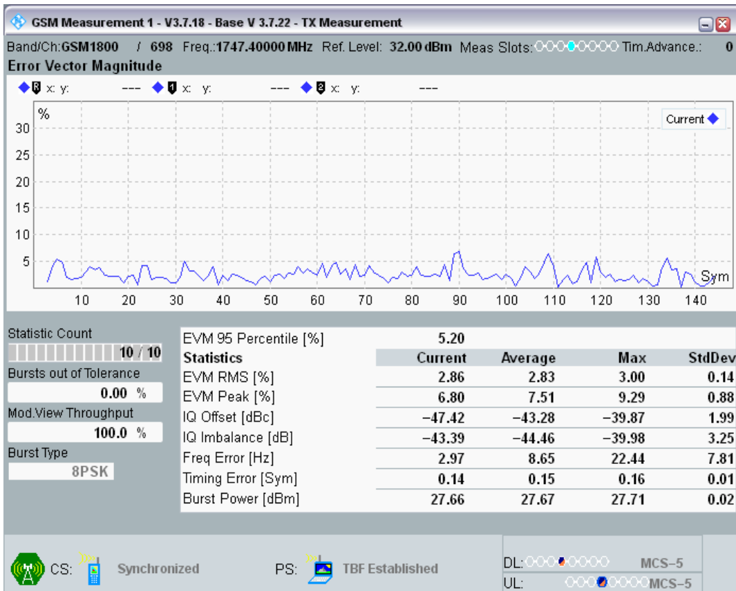
EGPRS1800 Channel=698 Gamma=5;5;5;5 TU3 @1
