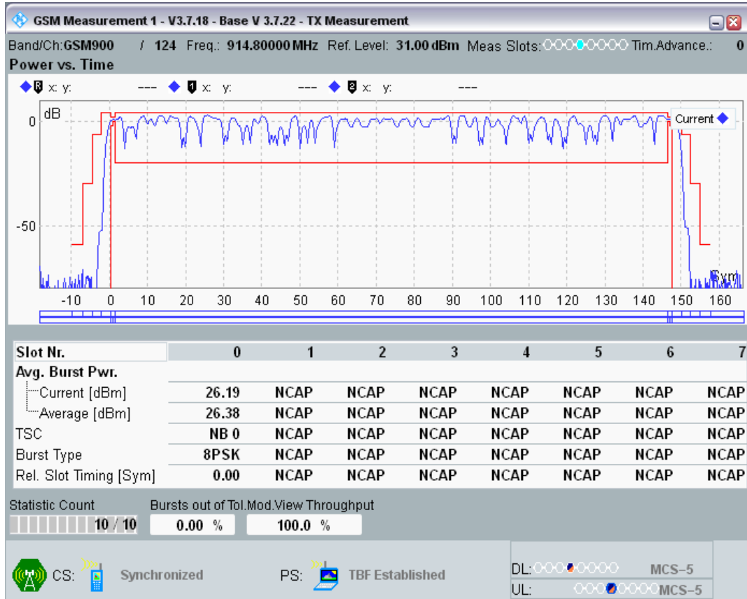
EGPRS900 Channel=124 Gamma=8;8;8;8
