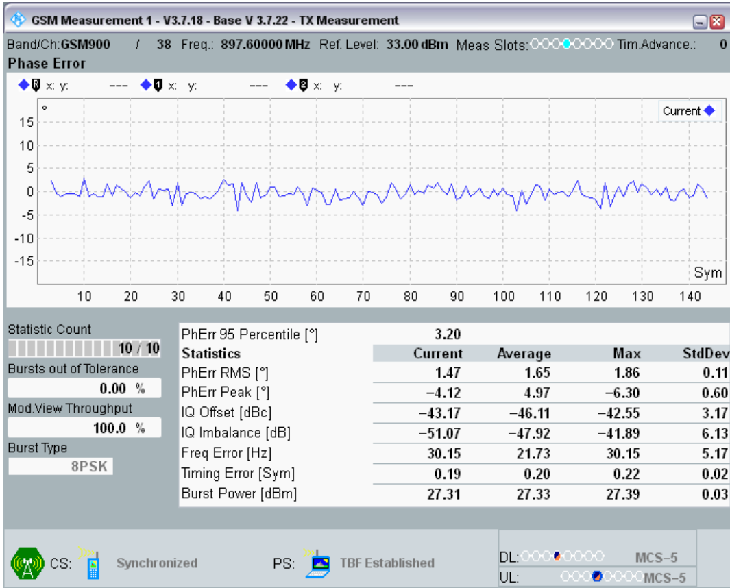
EGPRS900 Channel=38 Gamma=6;6;6;6 HT100 @Connect
