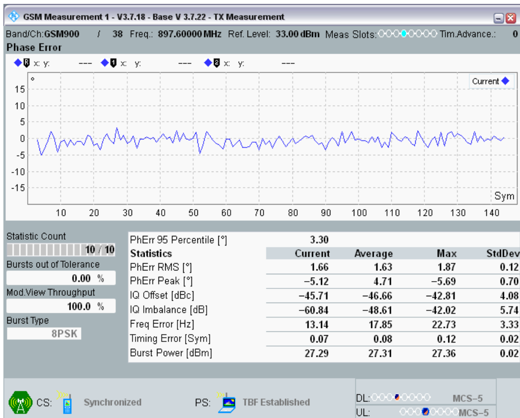
EGPRS900 Channel=38 Gamma=6;6;6;6 TU3 @19
