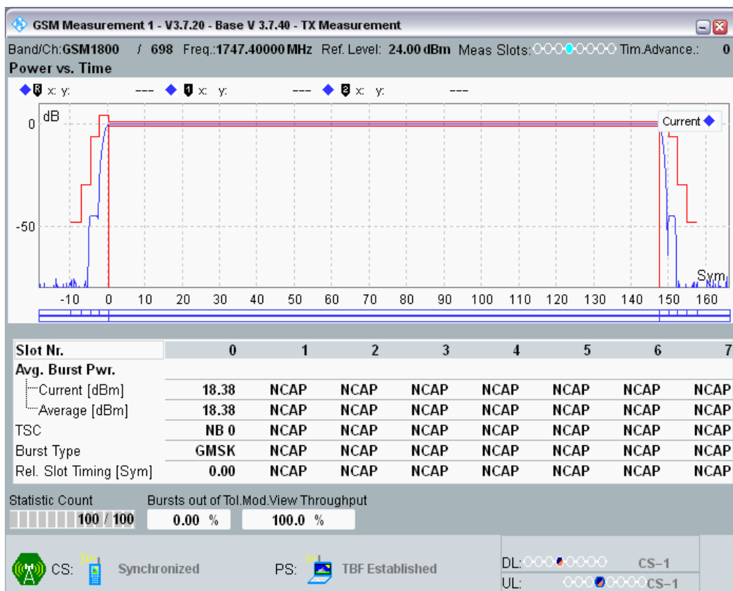
GPRS1800 Channel=698 Gamma=8;8;8;8
