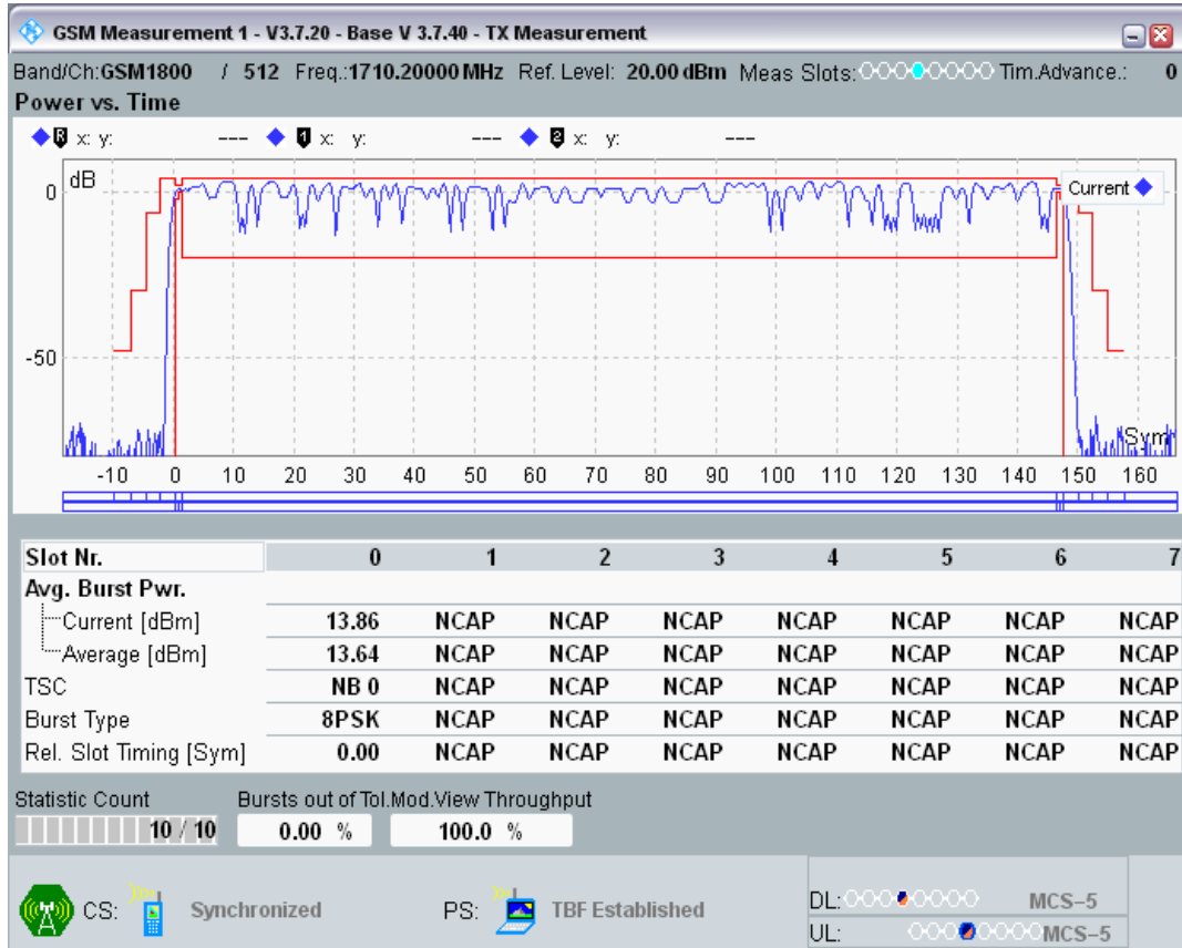
EGPRS1800 Channel=512 Gamma=10;10;10;10
