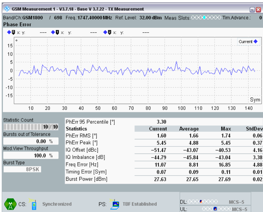
EGPRS1800 Channel=698 Gamma=5;5;5;5 TU3 @15
