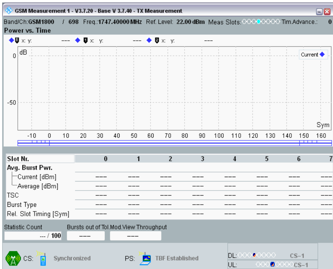
GPRS1800 Channel=512 Gamma=9;9;9;9
