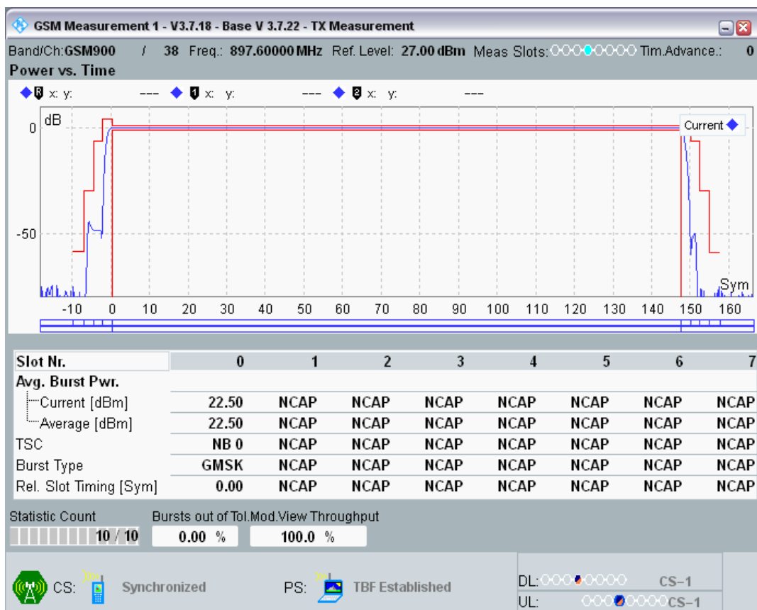
GPRS900 Channel=38 Gamma=10;10;10;10
