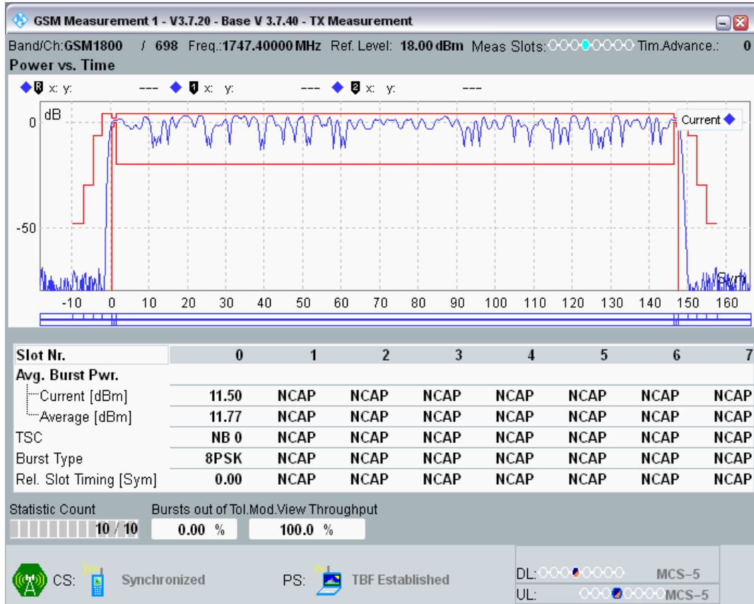
EGPRS1800 Channel=698 Gamma=13;13;13;13
