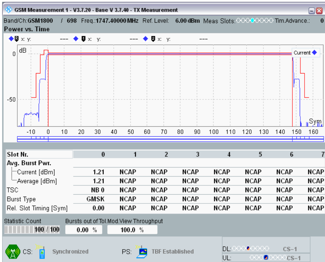
GPRS1800 Channel=698 Gamma=17;17;17;17
