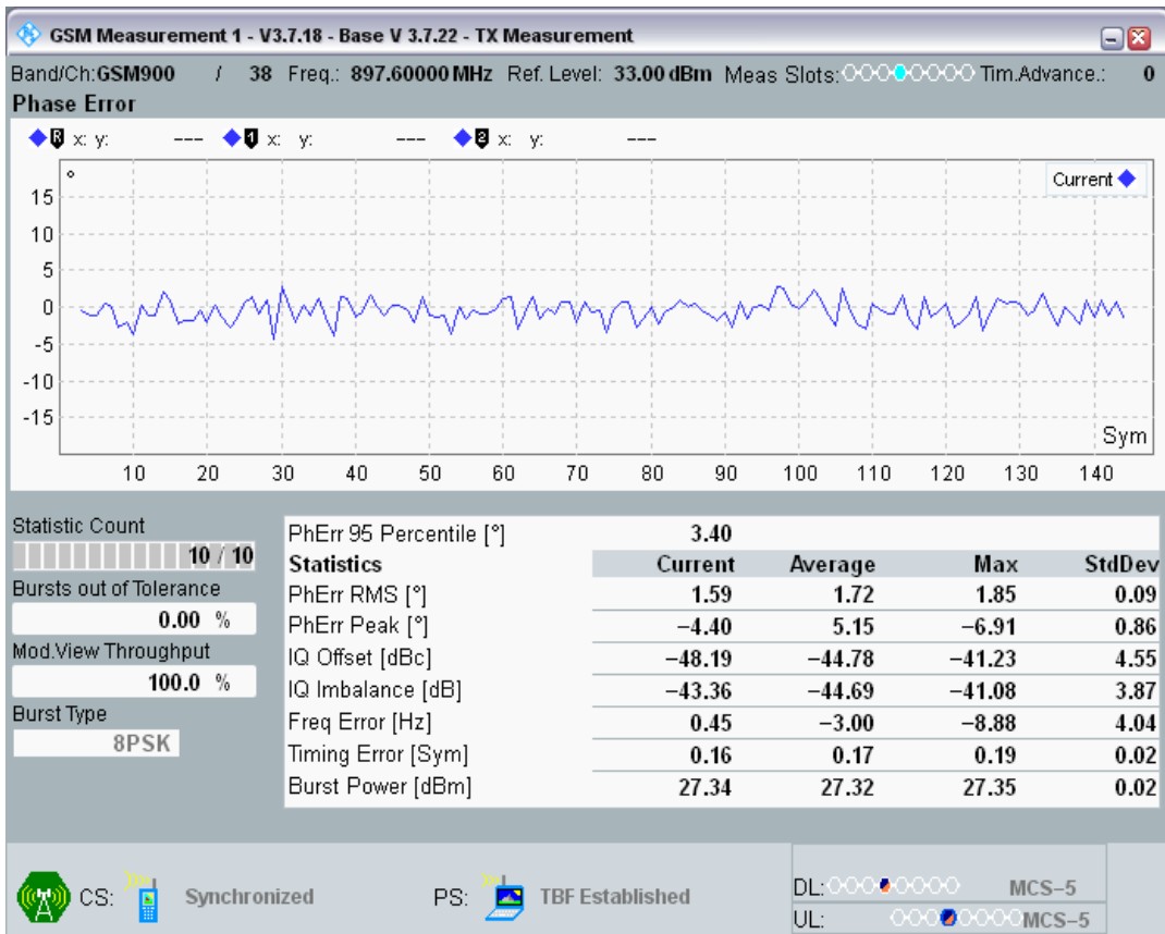
EGPRS900 Channel=38 Gamma=6;6;6;6 HT100 @Sens3
