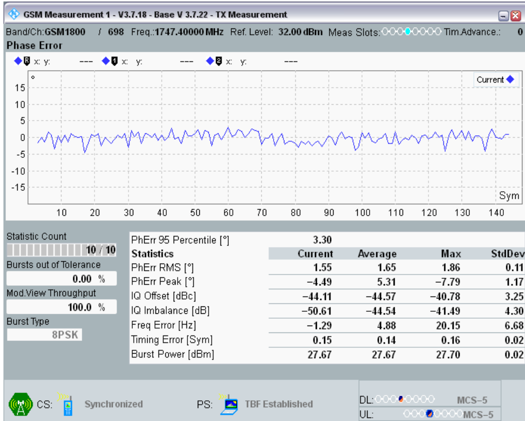
EGPRS1800 Channel=698 Gamma=5;5;5;5 TU3 @2
