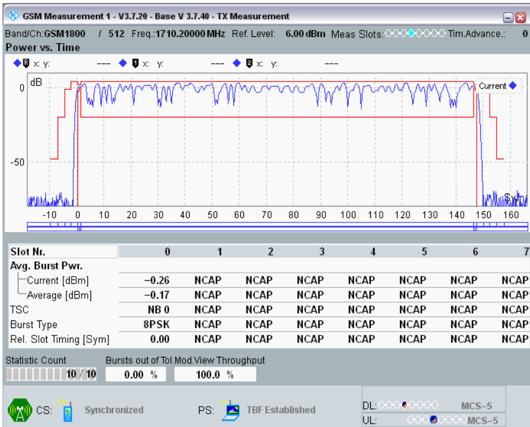
EGPRS1800 Channel=512 Gamma=11;11;11;11
