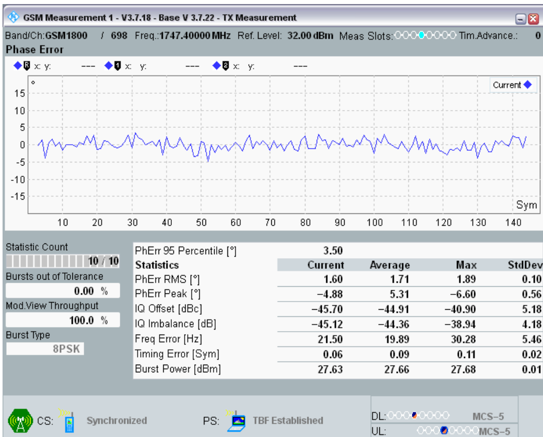
EGPRS1800 Channel=698 Gamma=5;5;5;5 TU3 @14
