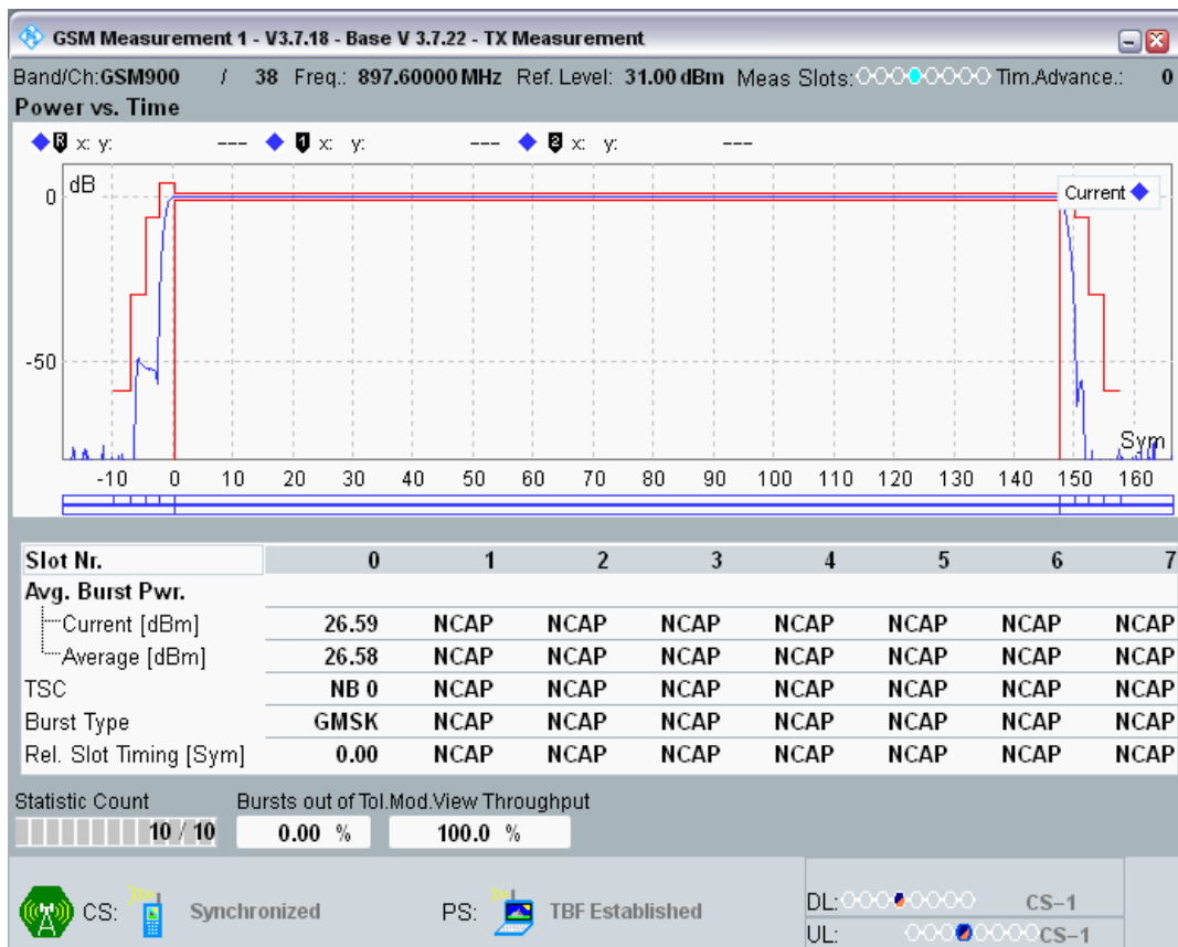
GPRS900 Channel=38 Gamma=8;8;8
