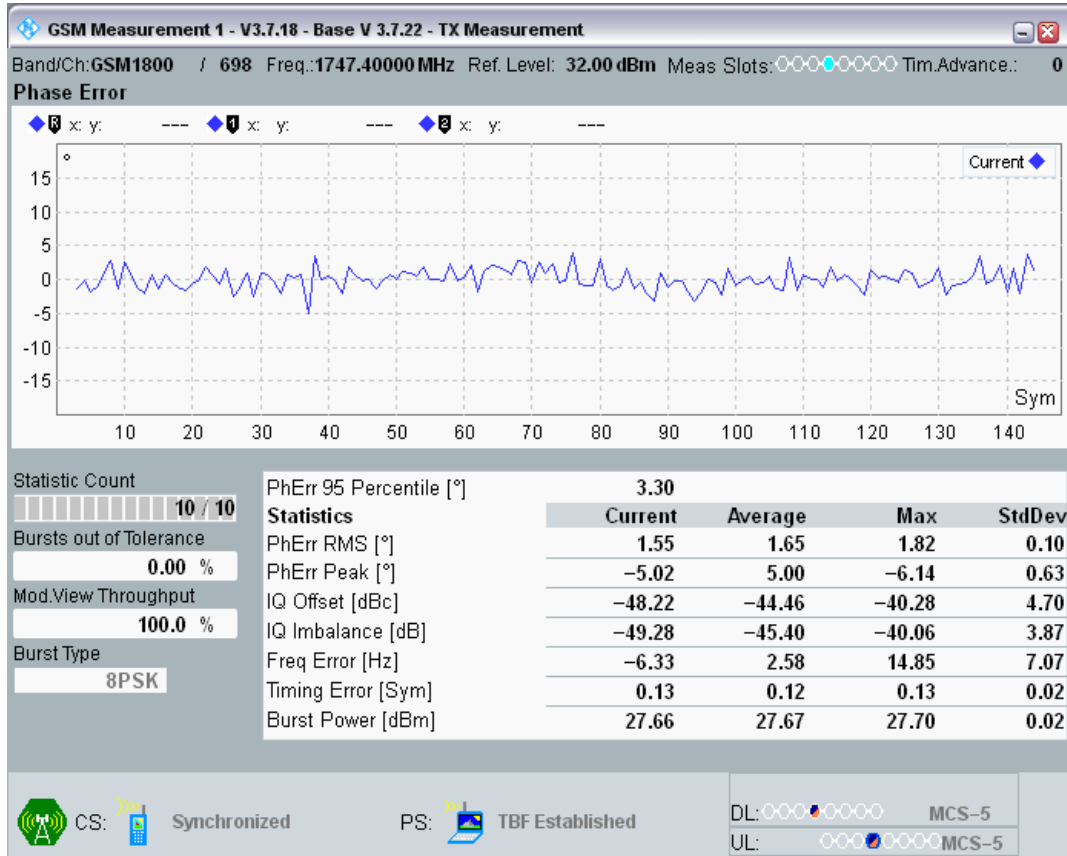
EGPRS1800 Channel=698 Gamma=5;5;5;5 TU3 @5
