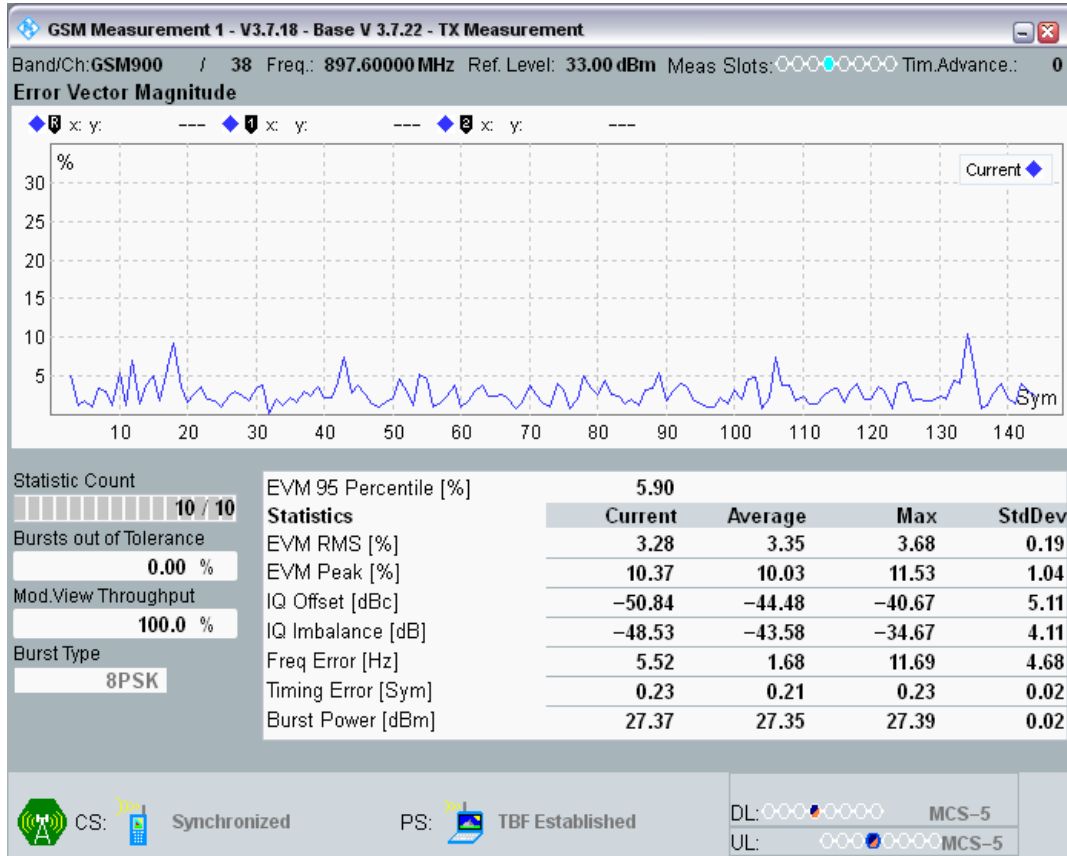
EGPRS900 Channel=38 Gamma=6;6;6;6 RA250 @Sens2
