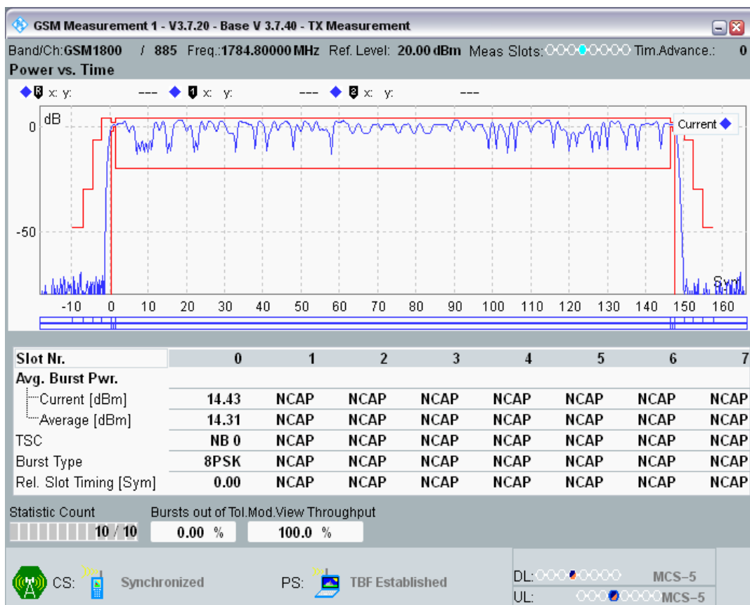
EGPRS1800 Channel=885 Gamma=10;10;10;10
