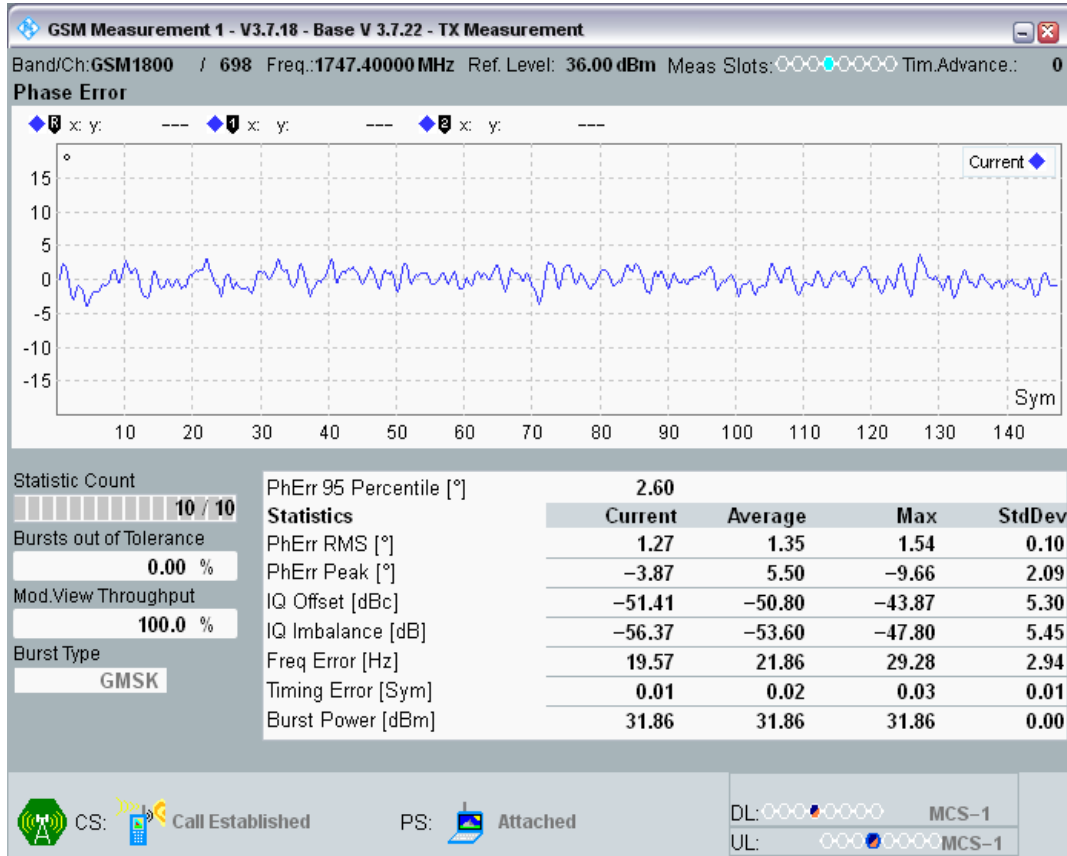
GSM1800 Channel=698 PCL=0 RA130 @Sens1
