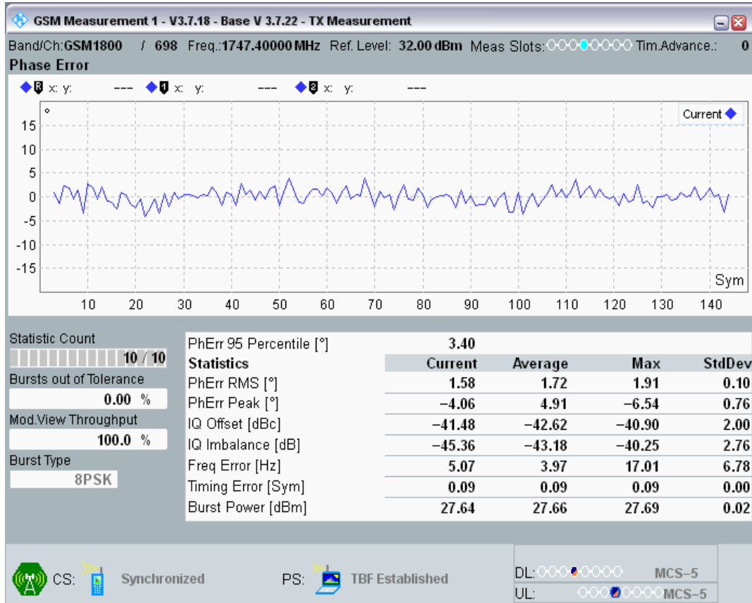
EGPRS1800 Channel=698 Gamma=5;5;5;5 TU3 @16
